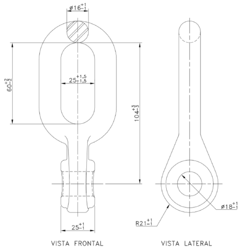
Figura 1 – Elo-Olhal 90°
