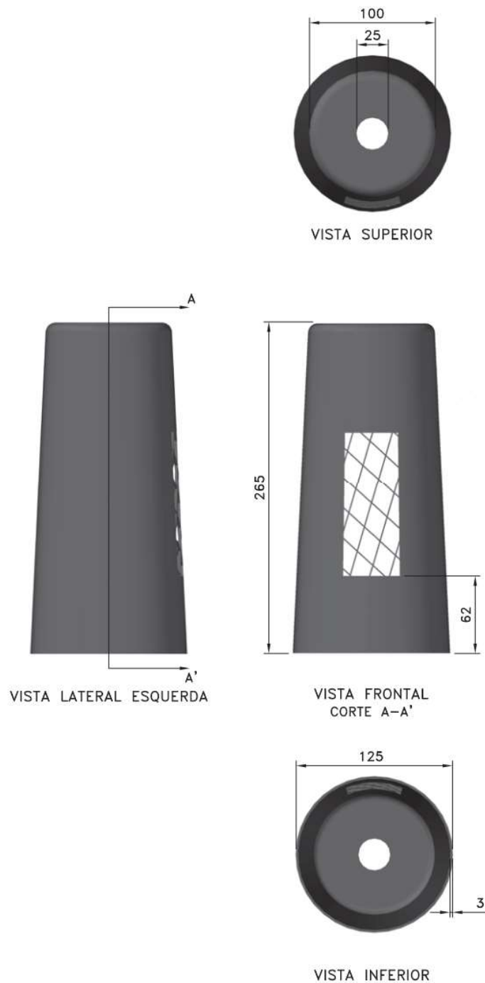
Figura 1 – Protetor para religador
