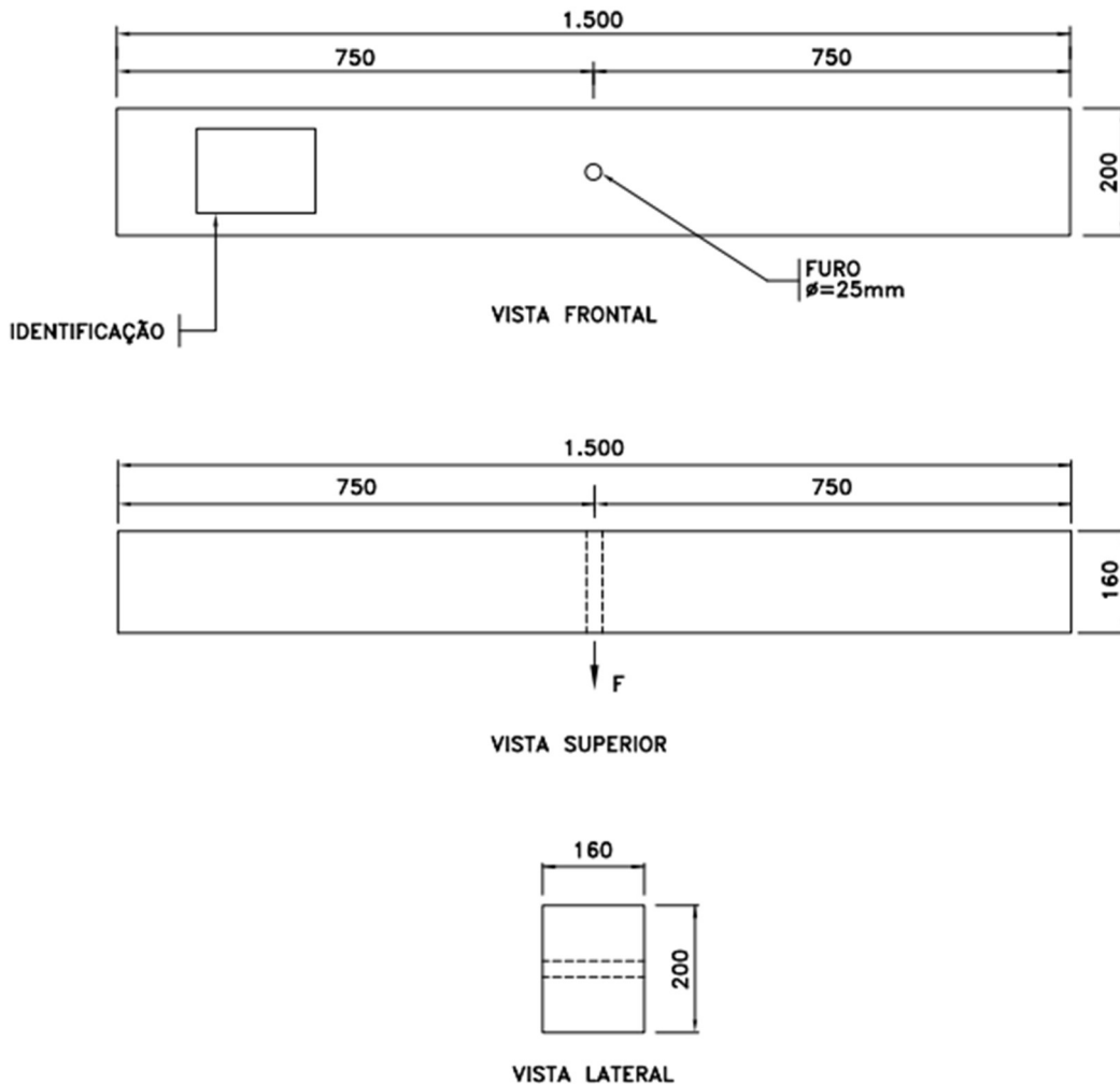
Figura 1 - Bloco de concreto dimensões
