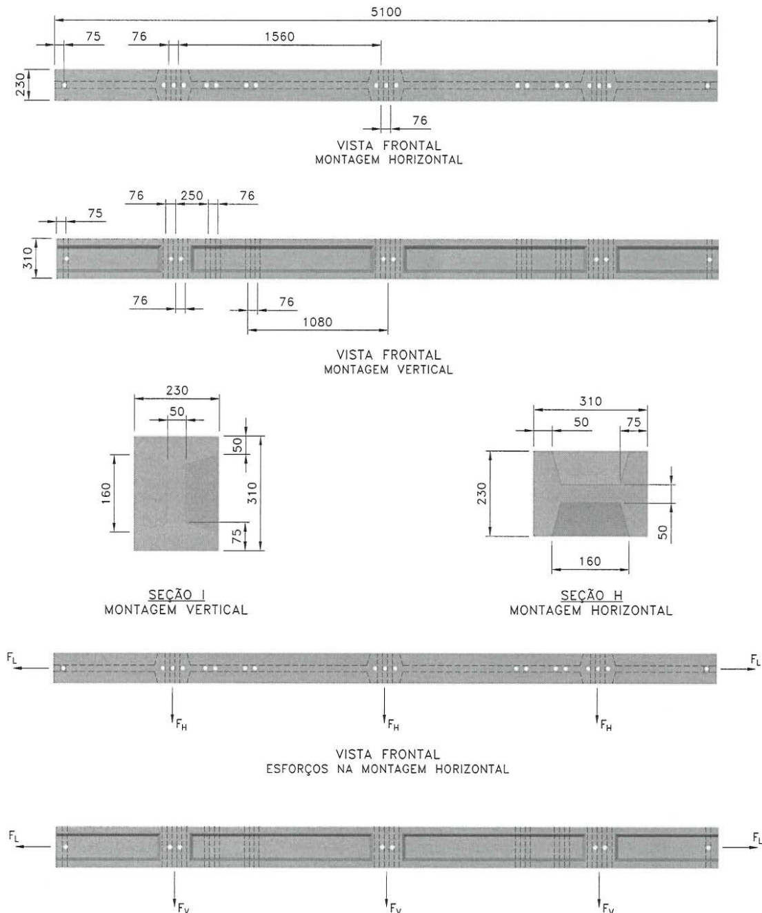
Figura 1 – Viga de Concreto Armado – Montagem Vertical e Horizontal
