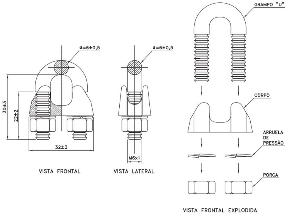
Figura 1 – Presilha em aço zincado
