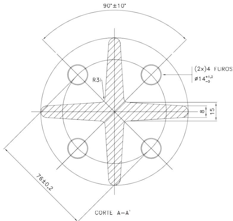
Figura 2 - Corte A-A
