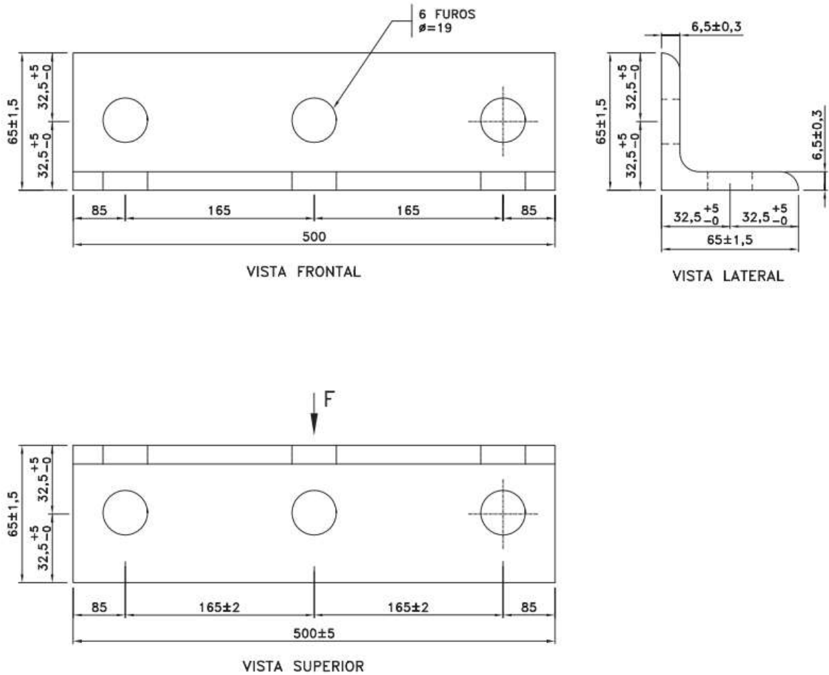
Figura 1 – Cantoneira perfil “L” em liga de alumínio
