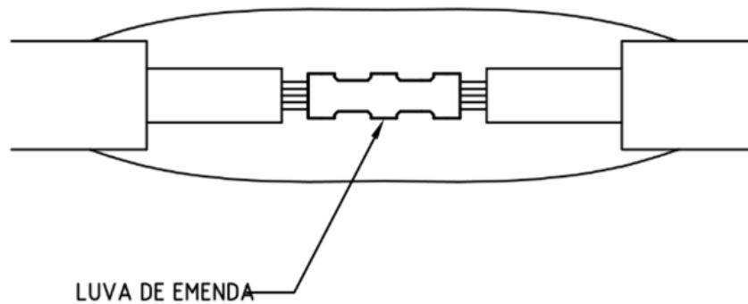
Figura 1 - Emenda reta para cabo de potência 0,6/1 kV monopolar
