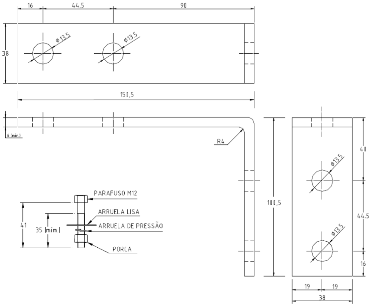
Figura 1 - Adaptador L para terminal
