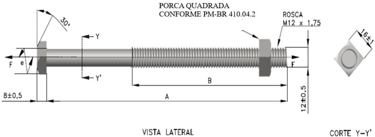
Figura 1 - Parafuso Cabeça Quadrada M12
