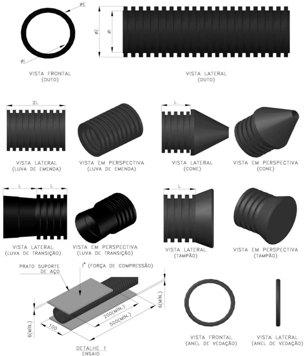
Figura 1 - Dutos Corrugados e Conexões
