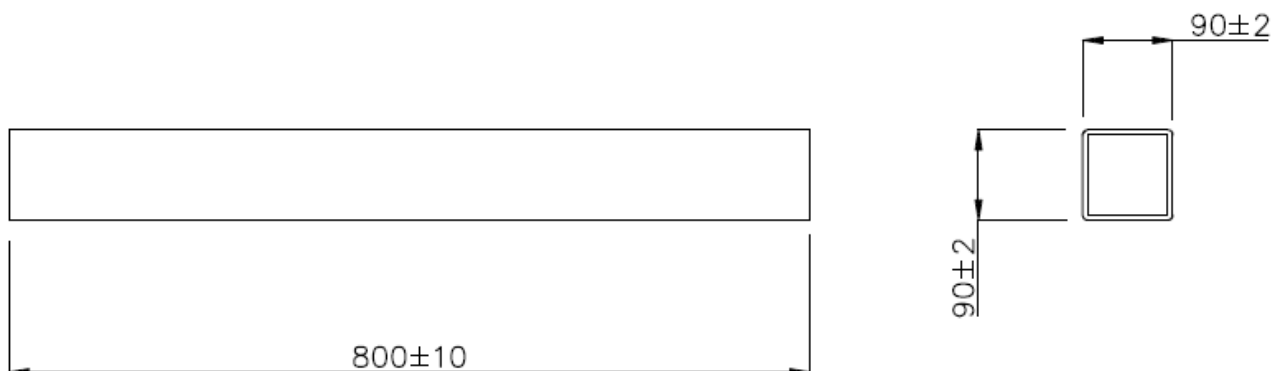
Figura 1 – Calço para Travar Postes
