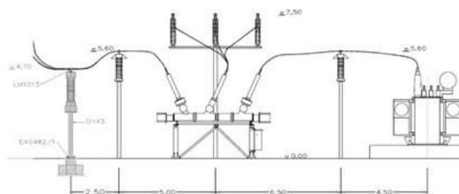
Figura 60 - Localização do transformador de potencial na seção AT (em cinza) no caso de módulo híbrido
