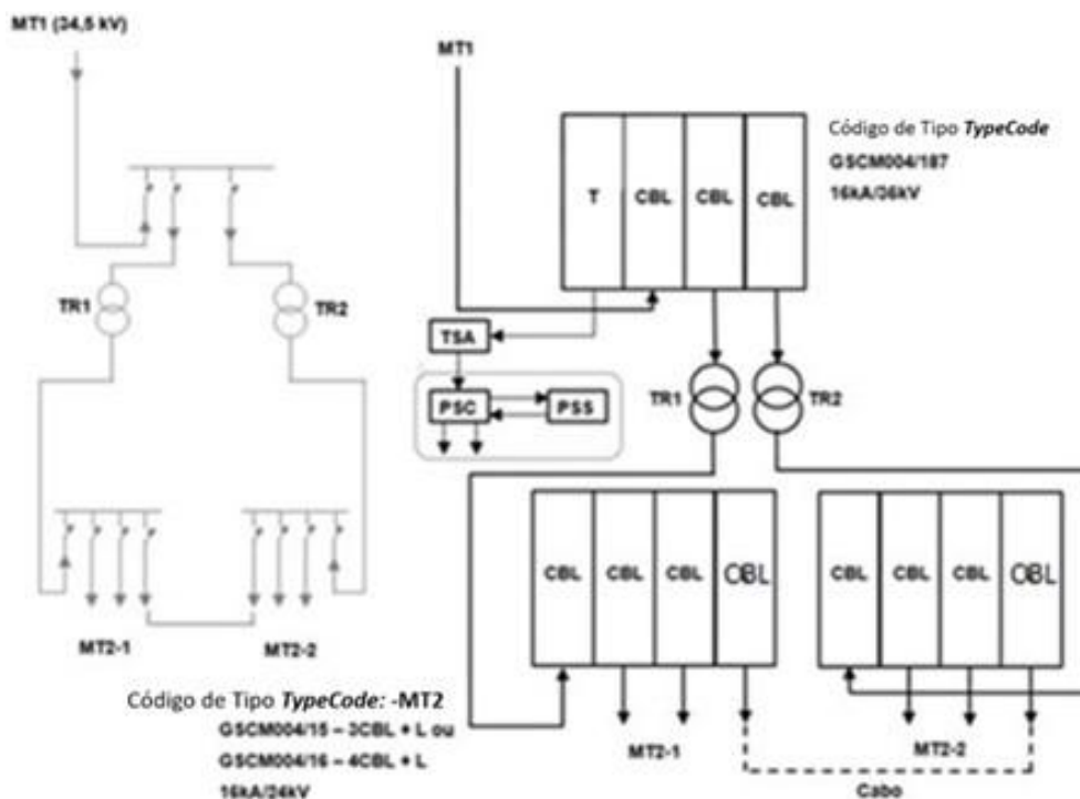
Figura 30 - Diagrama Subestação MT/MT - Tipo 2 (1 MT1 FINAL DE LINHA + 2T)
