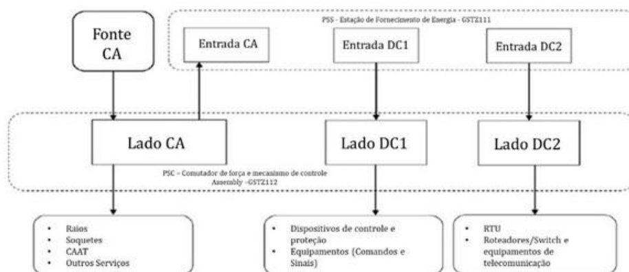
Figura 69 - Diagrama funcional da Estação de alimentação (PSS) e dos Serviços Auxiliares (PSC)
