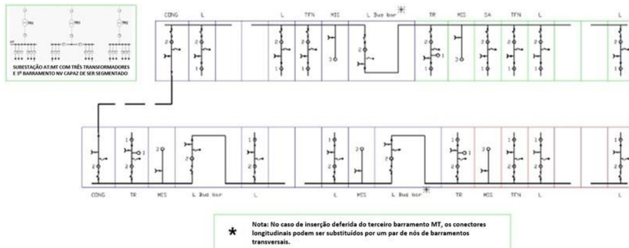
Figura 53 - GSCM009 na configuração de três transformadores
