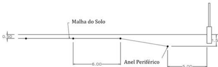
Figura 121 - Perfil da malha de solo
