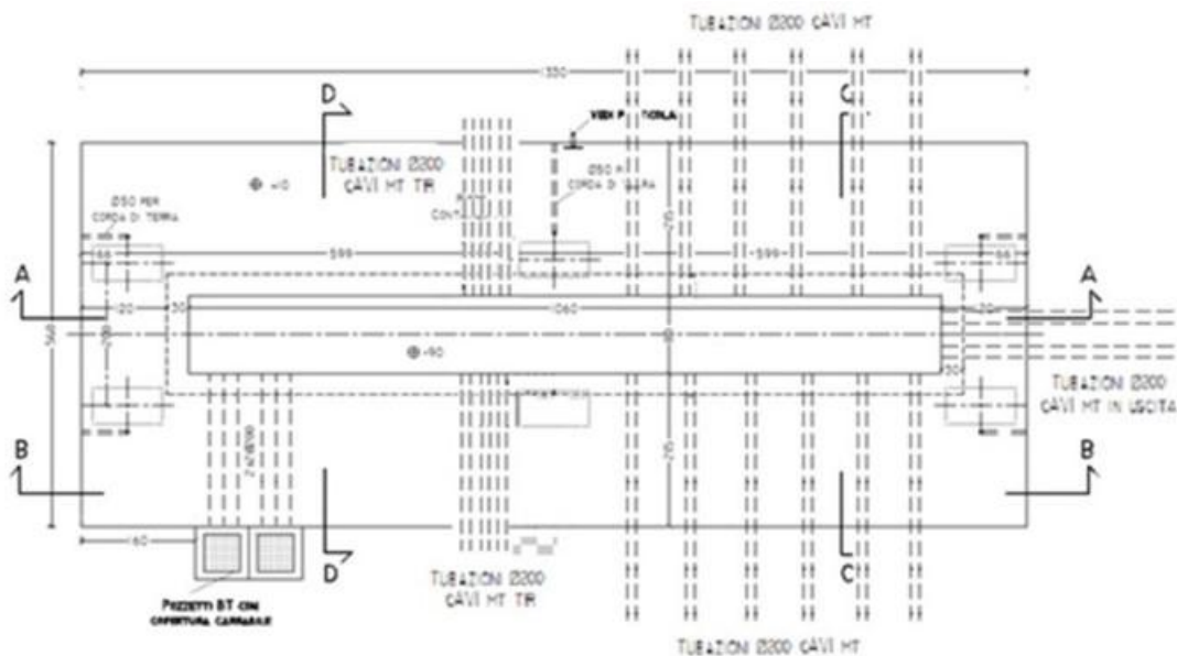
Figura 107 - Planta da fundação do container
