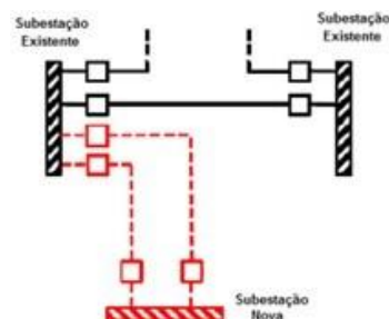
Figura 16 - Conexão Radial Dupla
