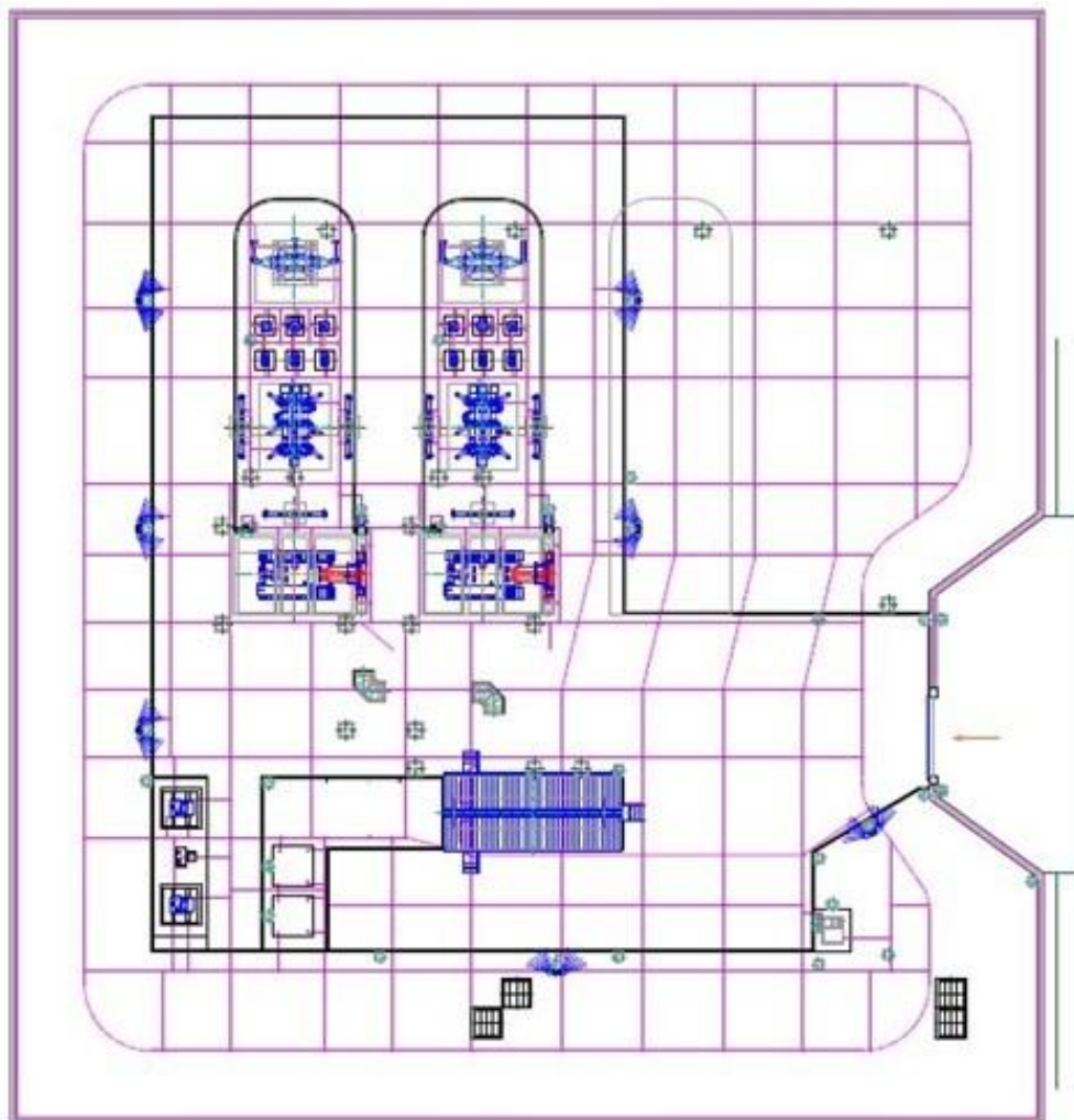
Figura 119 - Malha de Terra
