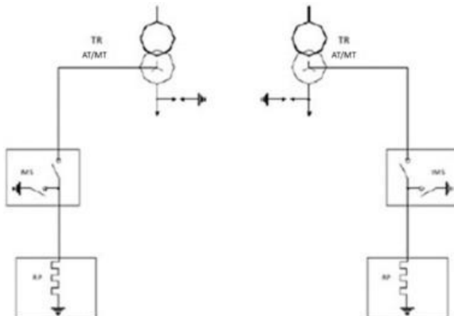
Figura 42 - Diagrama unifilar para conexão do resistor ao transformador AT/MT
