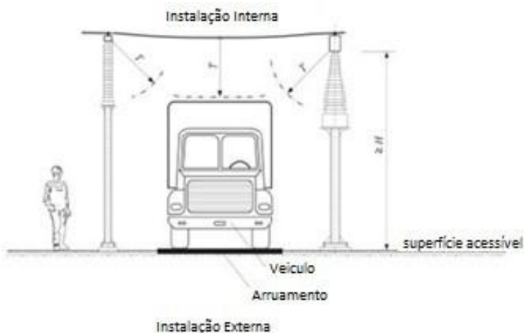
Figura 08 - Distância mínima de aproximação para transporte dentro de áreas elétricas de operação fechadas IEC - 61936
