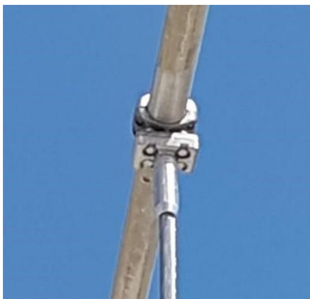
Figura 57 - Conexão de cabo \Phi 36mm ao tubo \Phi 100mm
