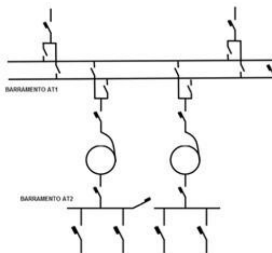
Figura 10 - Diagrama unifilar simplificado SED AT/AT com Função de Transformação
