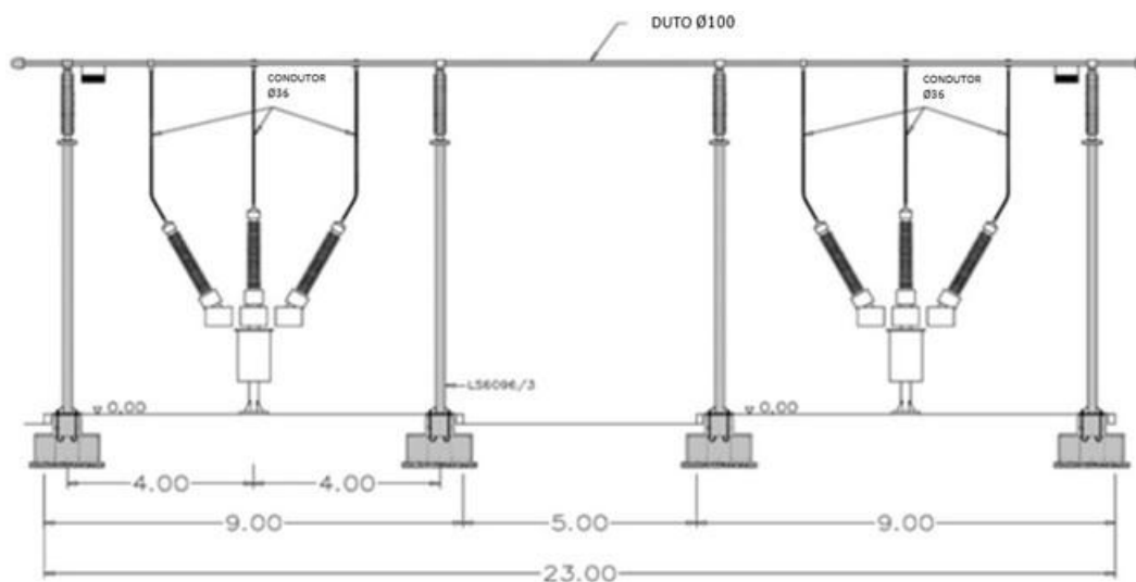
Figura 92 - Vista frontal do barramento principal de AT
