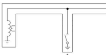
Figura 37 - Esquema do compartimento de barramento de medição
