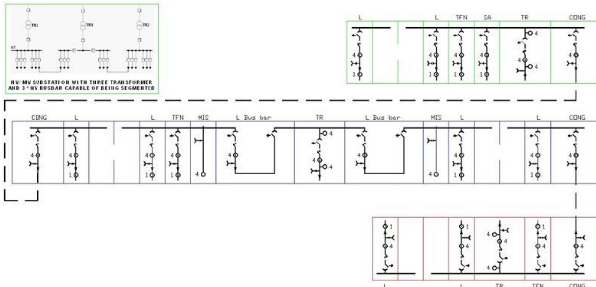
Figura 51 - GSCM011 na configuração de três transformadores com o barramento de 3ª MT passível de ser segmentado
