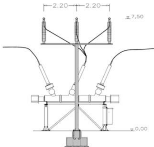
Figura 93 - Esquema de barramento AT (vista lateral esquerda)
