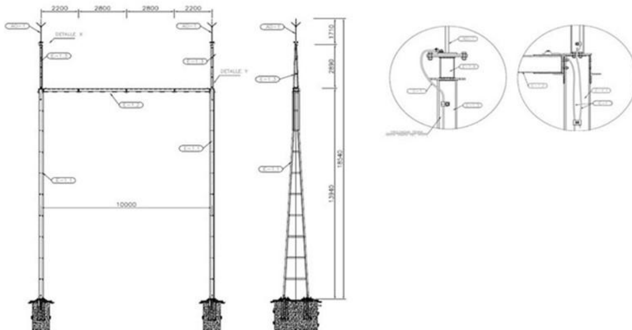
Figura 33 - Vista lateral e frontal da estrutura do pórtico AT
