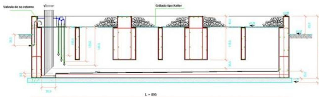
Figura 101 - Exemplo de base e recipiente de óleo único para dois transformadores AT/MT
