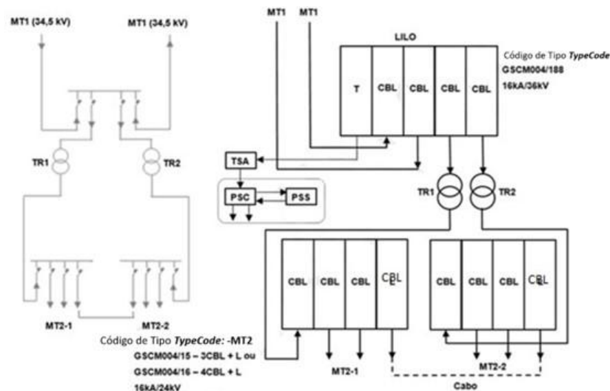
Figura 29 - Diagrama Subestação MT/MT - Tipo 2 (2 MT1 + 2T)
