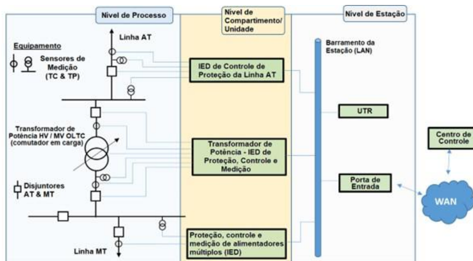
Figura 123 - Configuração do Sistema de Proteção e Controle de Subestações
