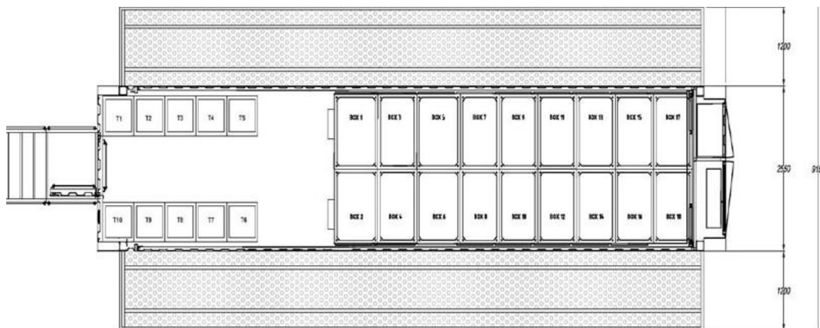
Figura 66 - Localização física dos dispositivos no container
