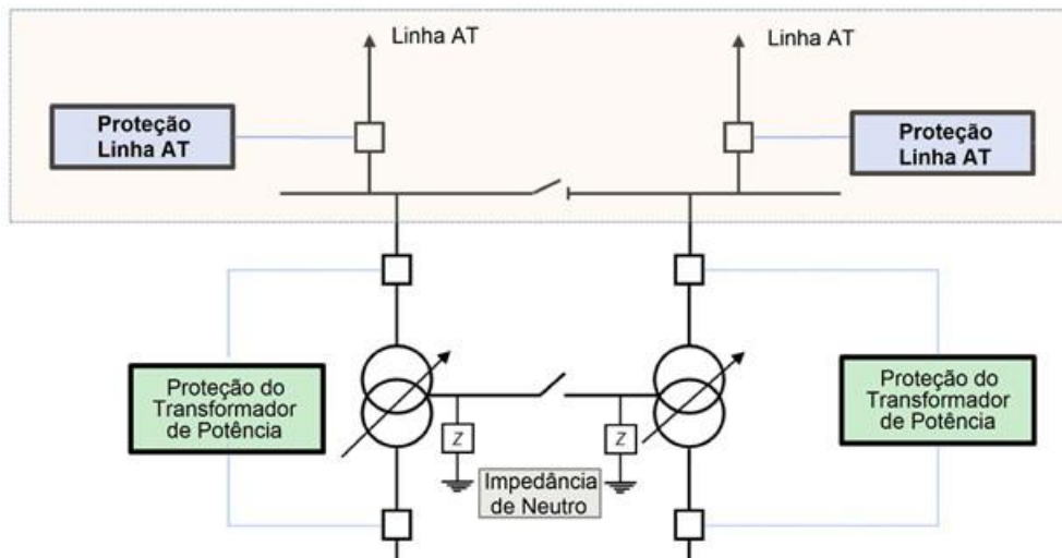
Figura 126 - Zonas de Proteção das Entradas e Saídas de Linha de AT
