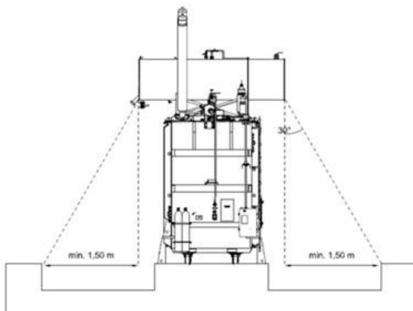
Figura 98 - Elevação da fundação do transformador
