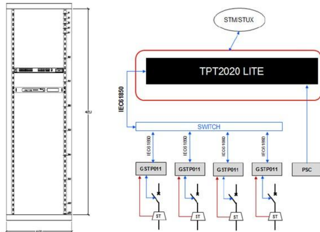
Figura 130 - Armário/Gabinete TPT 2020 Lite
