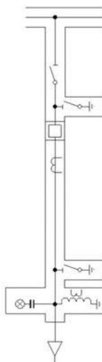
Figura 34 - Esquema do compartimento do transformador
