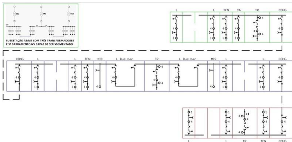
Figura 50 - GSCM011 na configuração de dois transformadores
