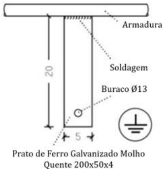
Figura 78 - Conexões de aterramento das fundações
