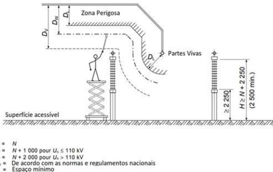
Figura 03 - Alturas e folgas mínimas de trabalho dentro de áreas de operação elétrica fechadas IEC – 61936
