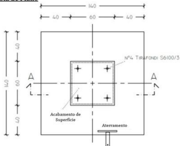
Figura 85 - Vista em planta da fundação unipolar
