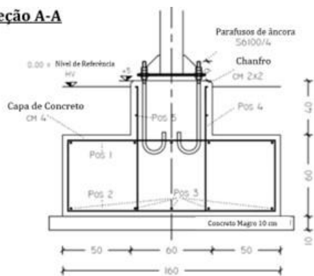
Figura 89 - Seção de fundação tripolar
