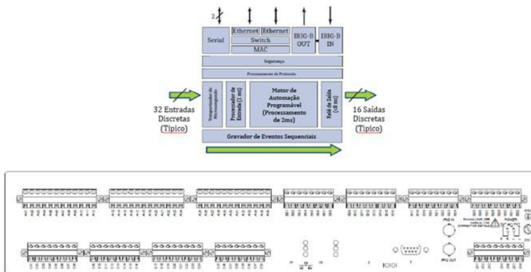
Figura 128 - Painel e Diagrama Funcional
