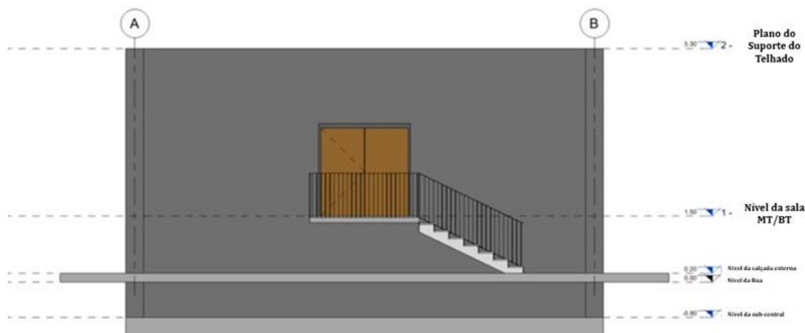
Figura 111 - Foco nos níveis do prédio em alvenaria da subestação
