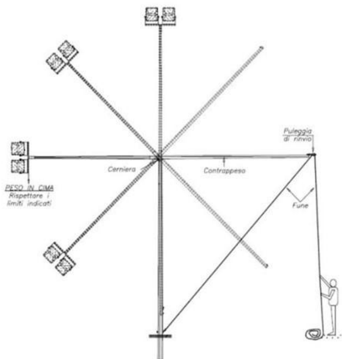
Figura 118 - Movimento do bastão basculante
