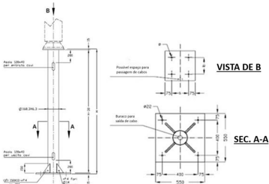
Figura 61 - Suporte de equipamento monopolar
