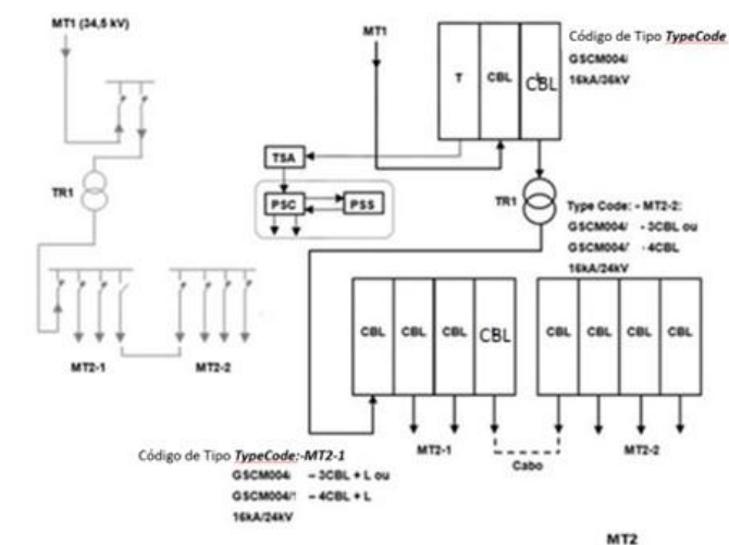
Figura 25 - Diagrama Subestação MT/MT - Tipo 1 (1 MT1 + 1T + até 6 MT2)
