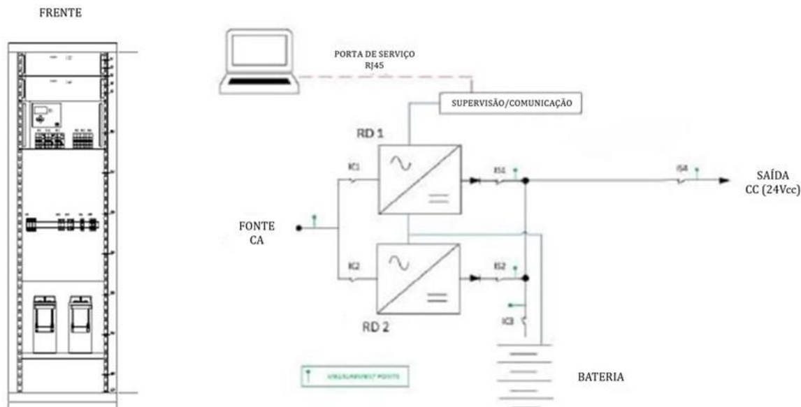
Figura 67 - Diagrama funcional e gabinete – Estação de alimentação (PSS)
