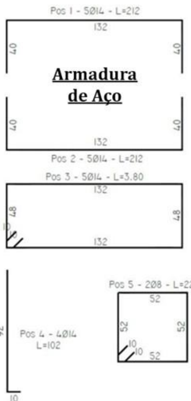
Figura 87 - Exemplo de projeto de armadura de aço para fundação unipolar
