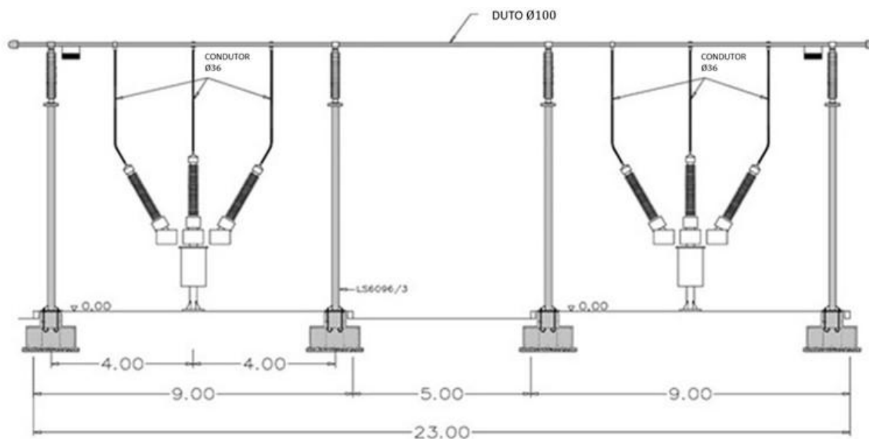
Figura 45 - Vista frontal do barramento principal de AT
