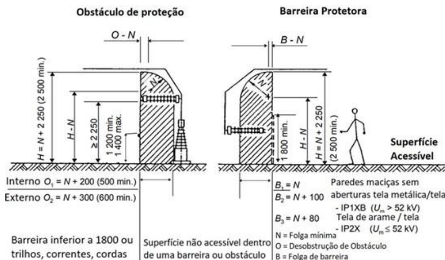
Figura 04 - Proteção contra contato direto por barreiras de proteção/obstáculos de proteção dentro de áreas de operação elétrica fechadas IEC – 61936
