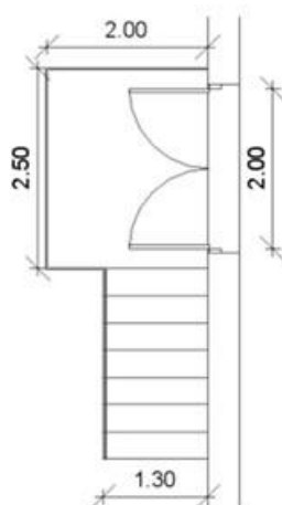
Figura 115 - Acessos principais às salas MT-BT
