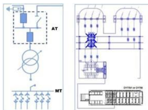
Figura 21 - Diagrama Subestação Simplificada LILO
