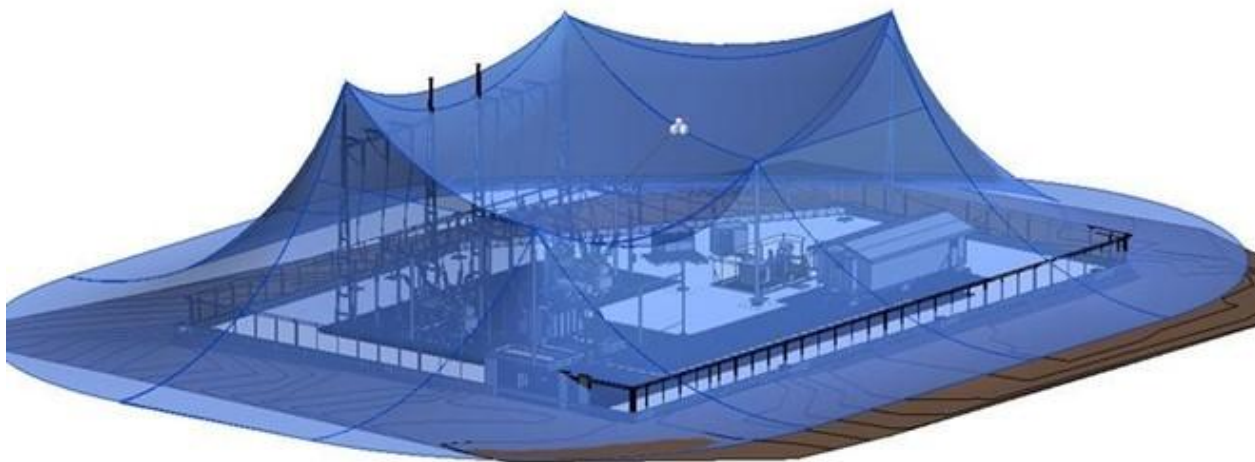
Figura 122 - Exemplo de área protegida pelo uso de hastes Franklin dentro da subestação
