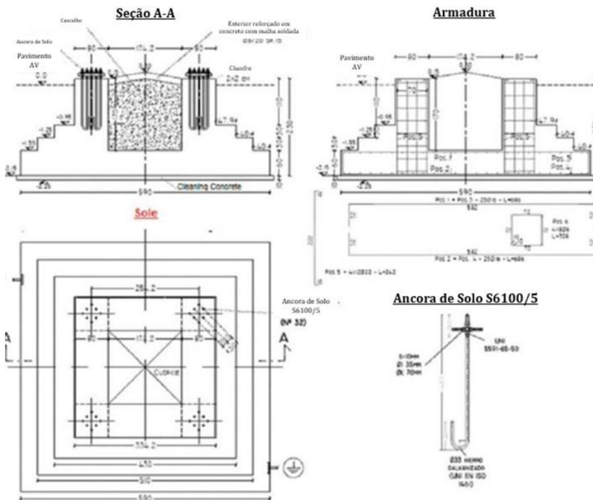
Figura 81 - Fundação Típica da Torre
