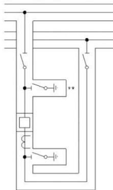
Figura 36 - Baía de acoplamento
