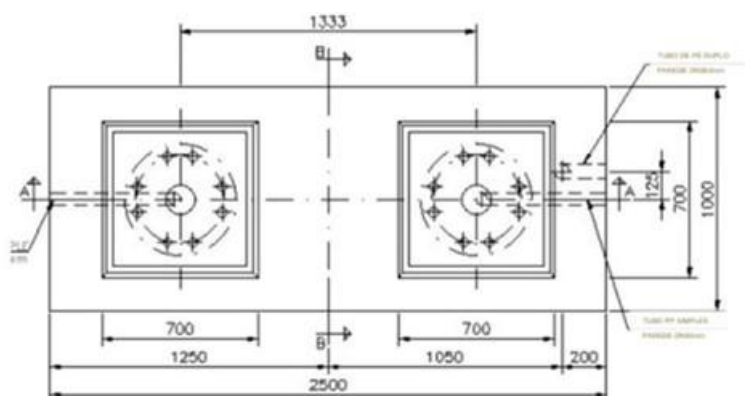
Figura 82 - Planta da Fundação da Torre Gantry
