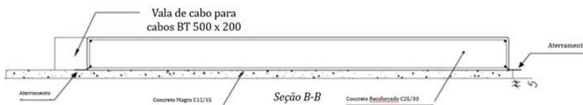
Figura 97 - Seção BB da Fundação do Módulo Híbrido
