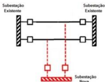
Figura 13 - Conexão em Derivação (Tap Dupla)
