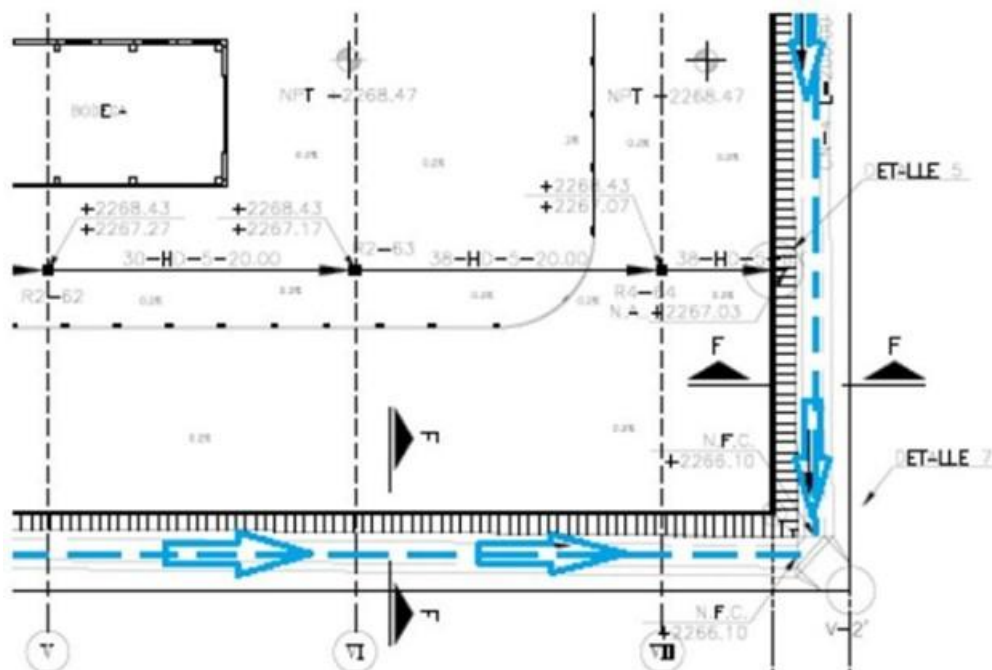
Figura 75 - Exemplo de planta que mostra as obras de drenagem da subestação plataforma e detalhe do ponto de descarga
