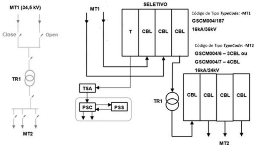
Figura 28 - Diagrama Subestação MT/MT Seletivo N-1
