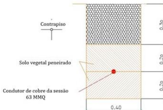
Figura 120 - Tipo de seção colocando malha principal
