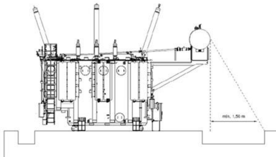
Figura 99 - Layout da fundação do transformador
