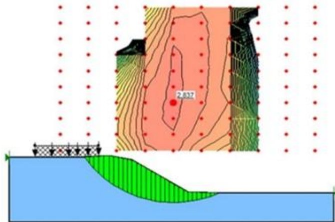
Figura 73 - Exemplo de verificação de estabilidade de talude
