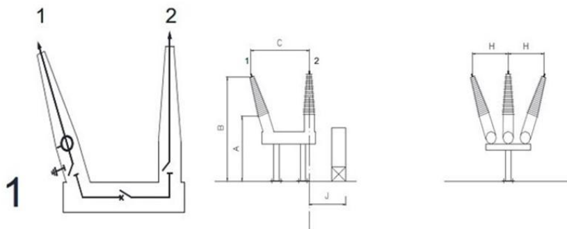
Figura 40 - Esquema elétrico, vista lateral e frontal do módulo de baía simples
