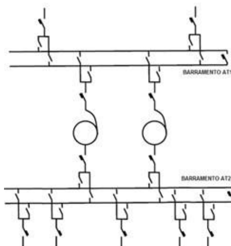
Figura 09 - Diagrama unifilar simplificado SED AT/AT com Função de Interface
