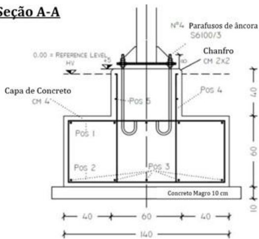
Figura 86 - Seção de fundação unipolar
