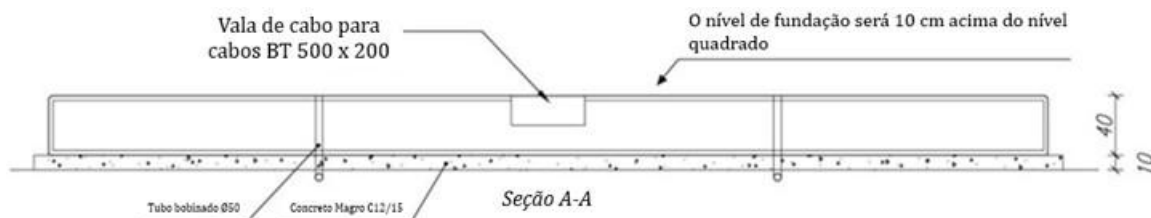
Figura 96 - Seção AA da Fundação do Módulo Híbrido
