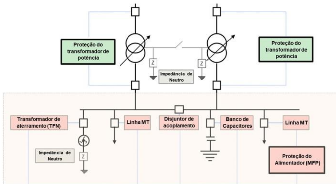
Figura 131 - Zonas de proteção MT
