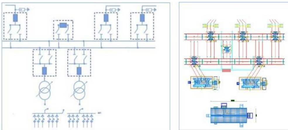
Figura 22 - Diagrama Subestação Especial Nodal
