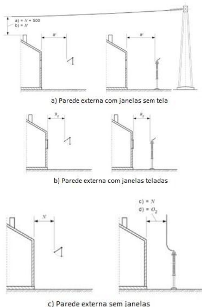
Figura 07 - Folga entre partes ativas e edificações IEC – 61936
