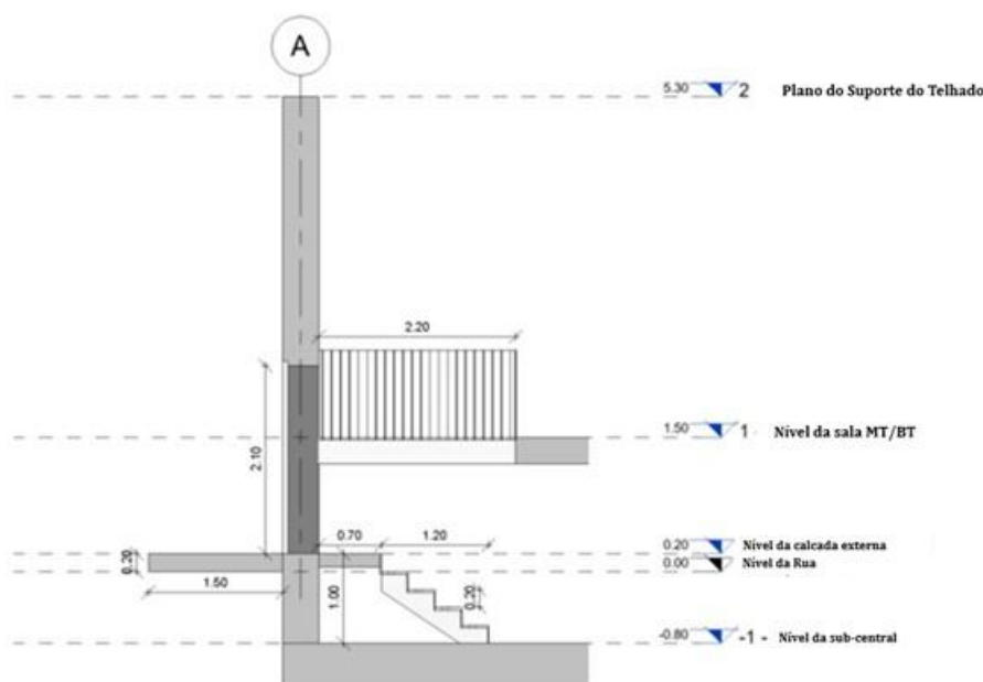
Figura 112 - Secção particular da escada de emergência da sub-central
