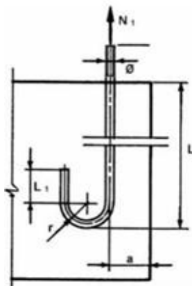
Figura 80 - Geometria típica dos chumbadores
