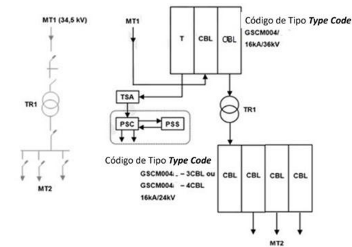
Figura 24 - Diagrama Subestação MT/MT - Tipo 1 (1 MT1 + 1T)
