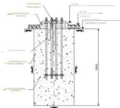
Figura 84 - Trecho BB da Pórtico Fundação
