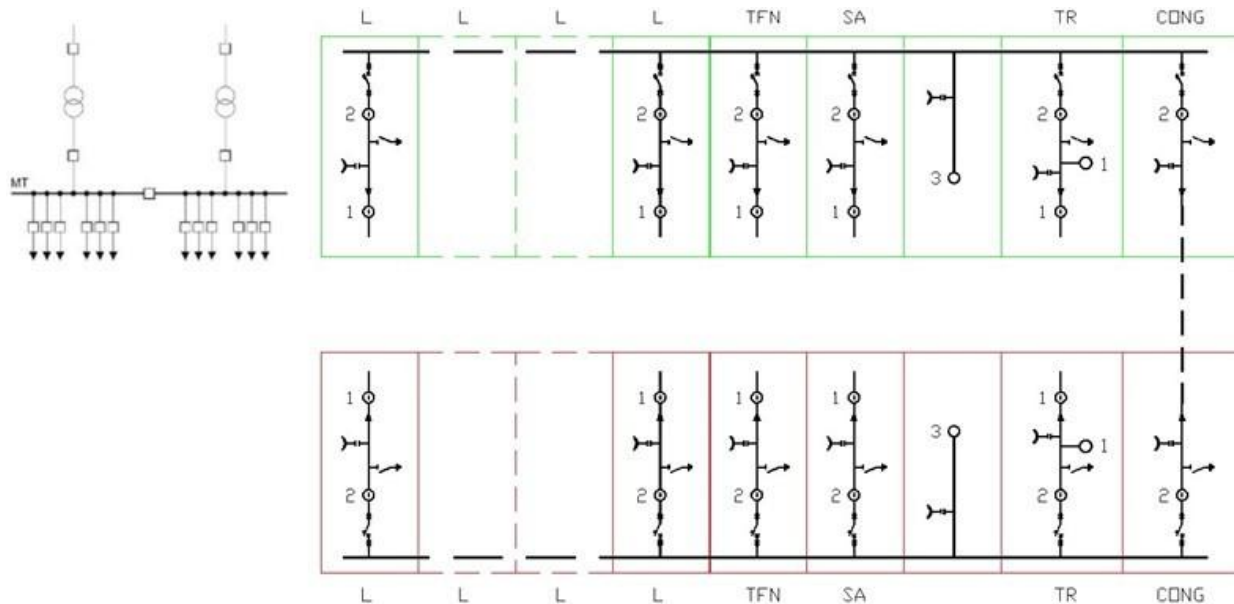
Figura 52 - GSCM009 na configuração de dois transformadores
