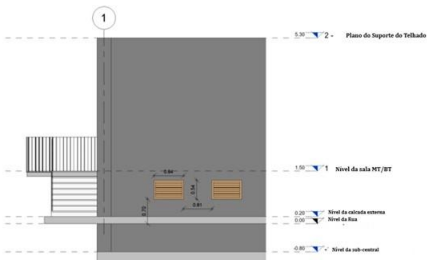
Figura 114 - Aberturas de ventilação do subquadro
