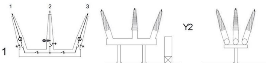
Figura 39 - Esquema elétrico, vista lateral e frontal do módulo Y2
