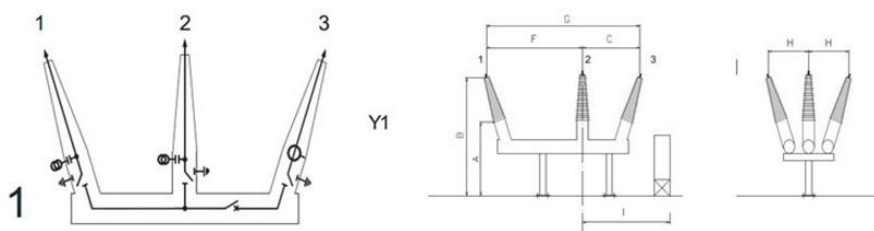
Figura 38 - Esquema elétrico, vista lateral e frontal do módulo Y1
