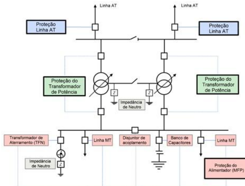
Figura 125 - Sistema de Proteção para Subestações AT/MT
