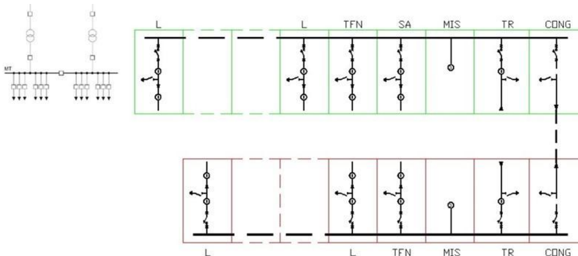
Figura 48 - GSCM690 na configuração de dois transformadores
