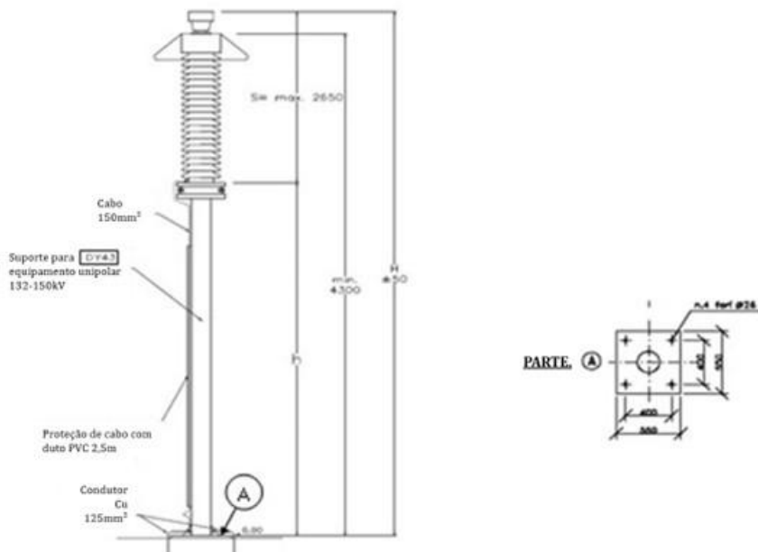
Figura 63 - Para-raios 132-150 kV
