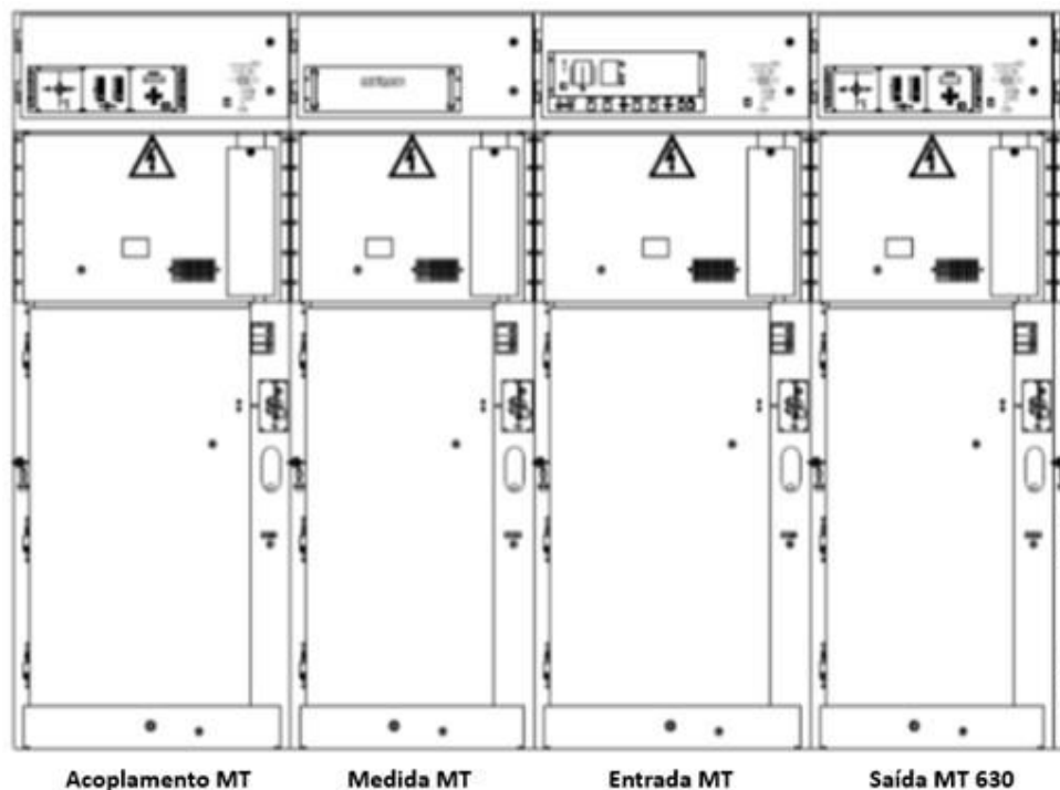
Figura 132 - Proteção e controle IED do transformador na linha de painéis de distribuição MT
