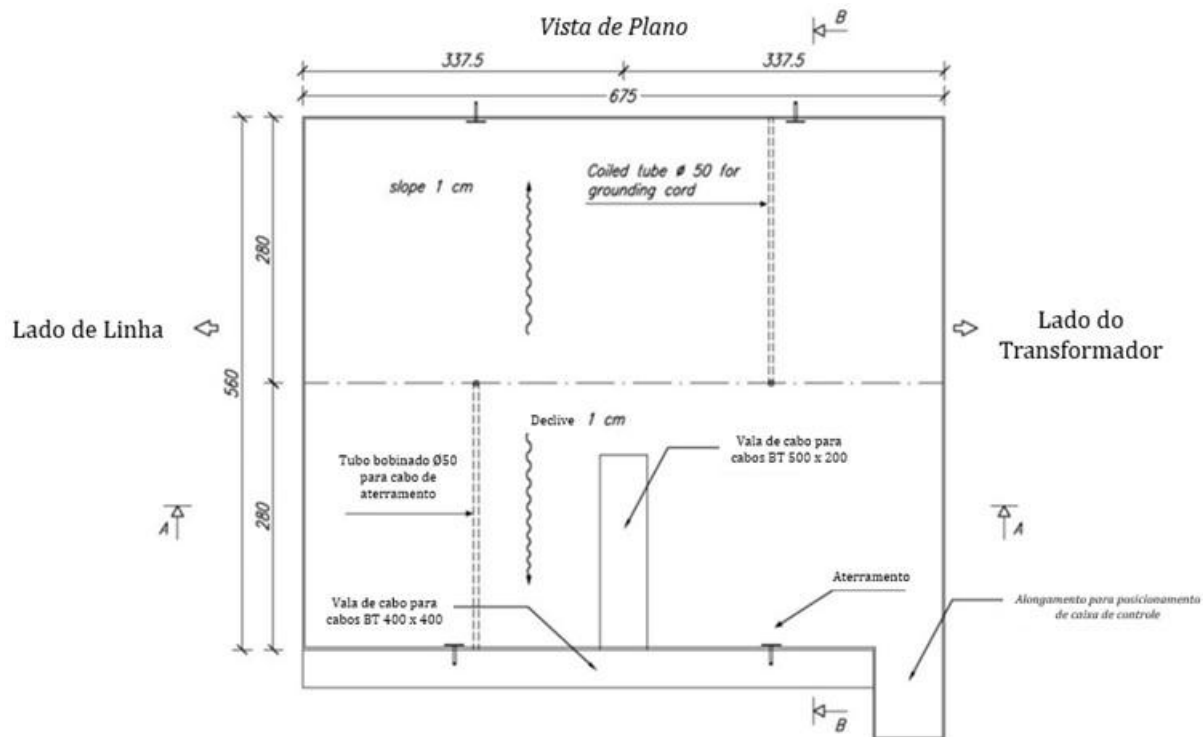
Figura 95 - Fundação detalhada do módulo híbrido Planview
