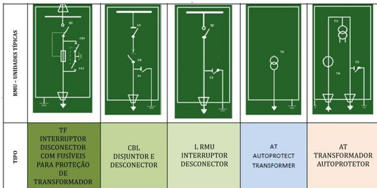
Figura 54 - Unidades funcionais – MT Switchgear GSCM004
