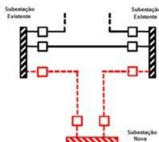
Figura 15 - Conexão LILLO de vãos (bays) novos
