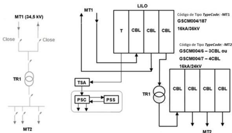
Figura 27 - Diagrama Subestação MT/MT LILO
