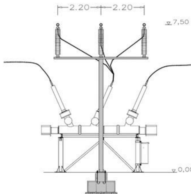
Figura 46 - Vista lateral esquerda e corte do barramento de alta tensão
