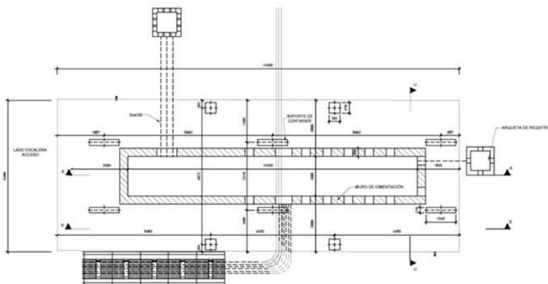
Figura 106 - Visão geral da fundação do container
