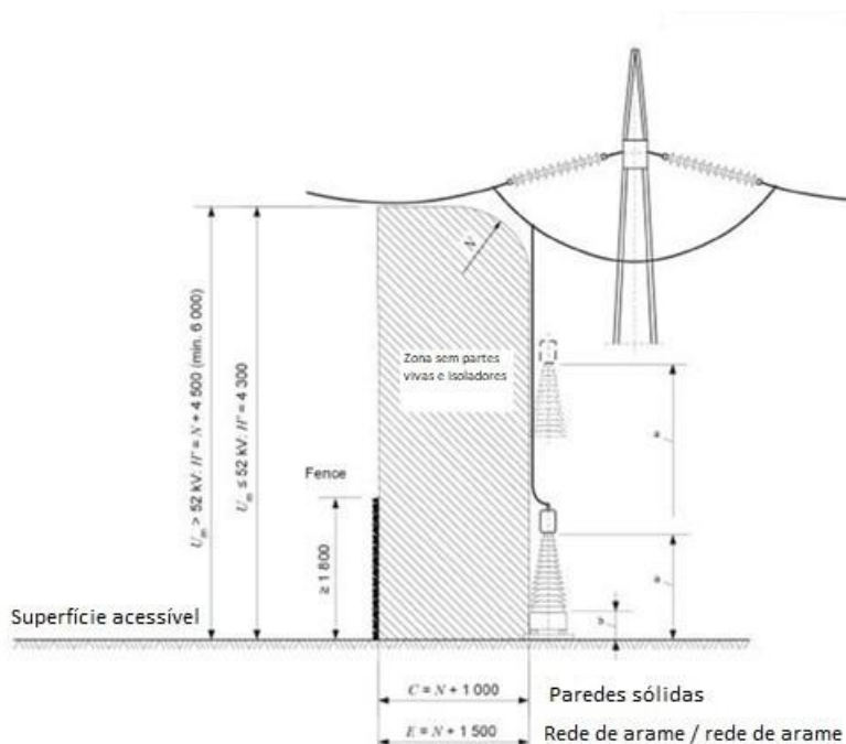
Figura 05 - Distâncias de limite e altura mínima até a cerca/parede externa IEC - 61936
