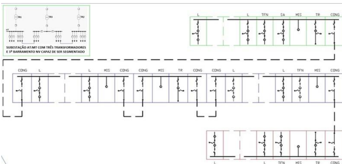
Figura 49 - GSCM690 na configuração de três transformadores com barramento de 3º MT capaz de ser segmentado
