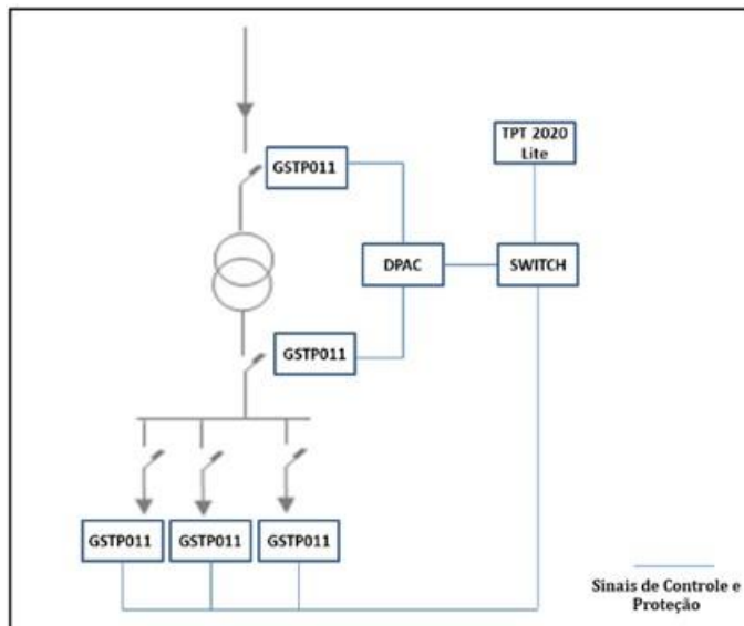
Figura 129 - Diagrama de proteção e controle da subestação
