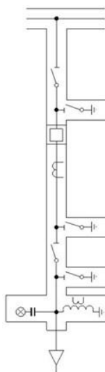
Figura 35 - Esquema de baias da Linha GIS
