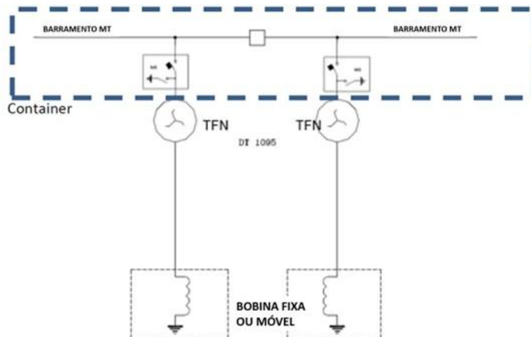
Figura 44 - Diagrama unifilar para neutro aterrado com TFN e bobina de Petersen
