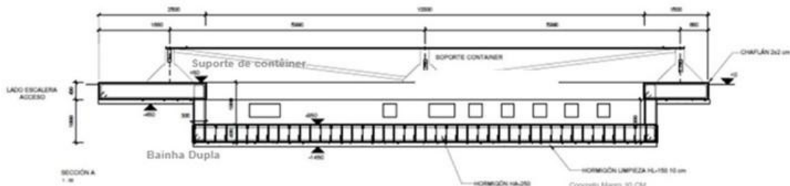
Figura 108 - Seção AA da fundação do container
