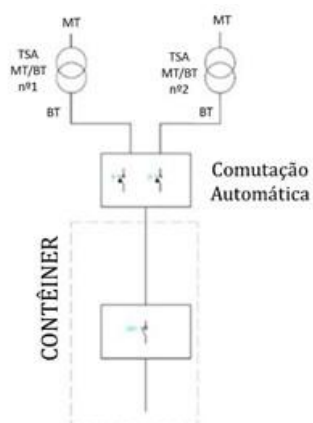
Figura 68 - Esquema de alimentação dos Serviços Auxiliares
