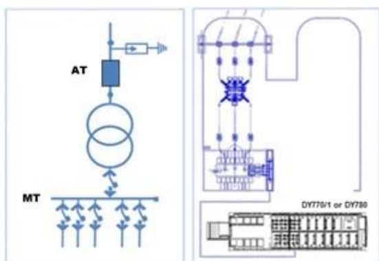
Figura 20 - Diagrama Subestação Simplificada Radial e TAP
