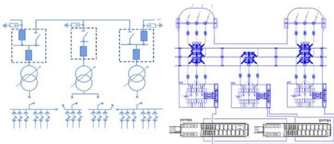
Figura 23 - Diagrama Subestação Especial com 3 Transformadores
