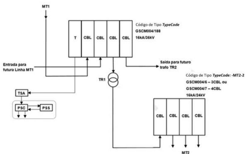
Figura 26 - Diagrama Subestação MT/MT para futura ampliação
