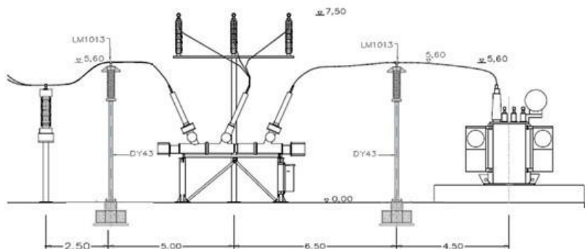
Figura 62 - Localização dos para-raios (em cinza) em combinação com o módulo híbrido
