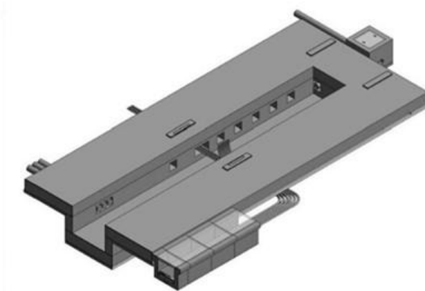
Figura 105 - Modelo 3D da fundação do container
