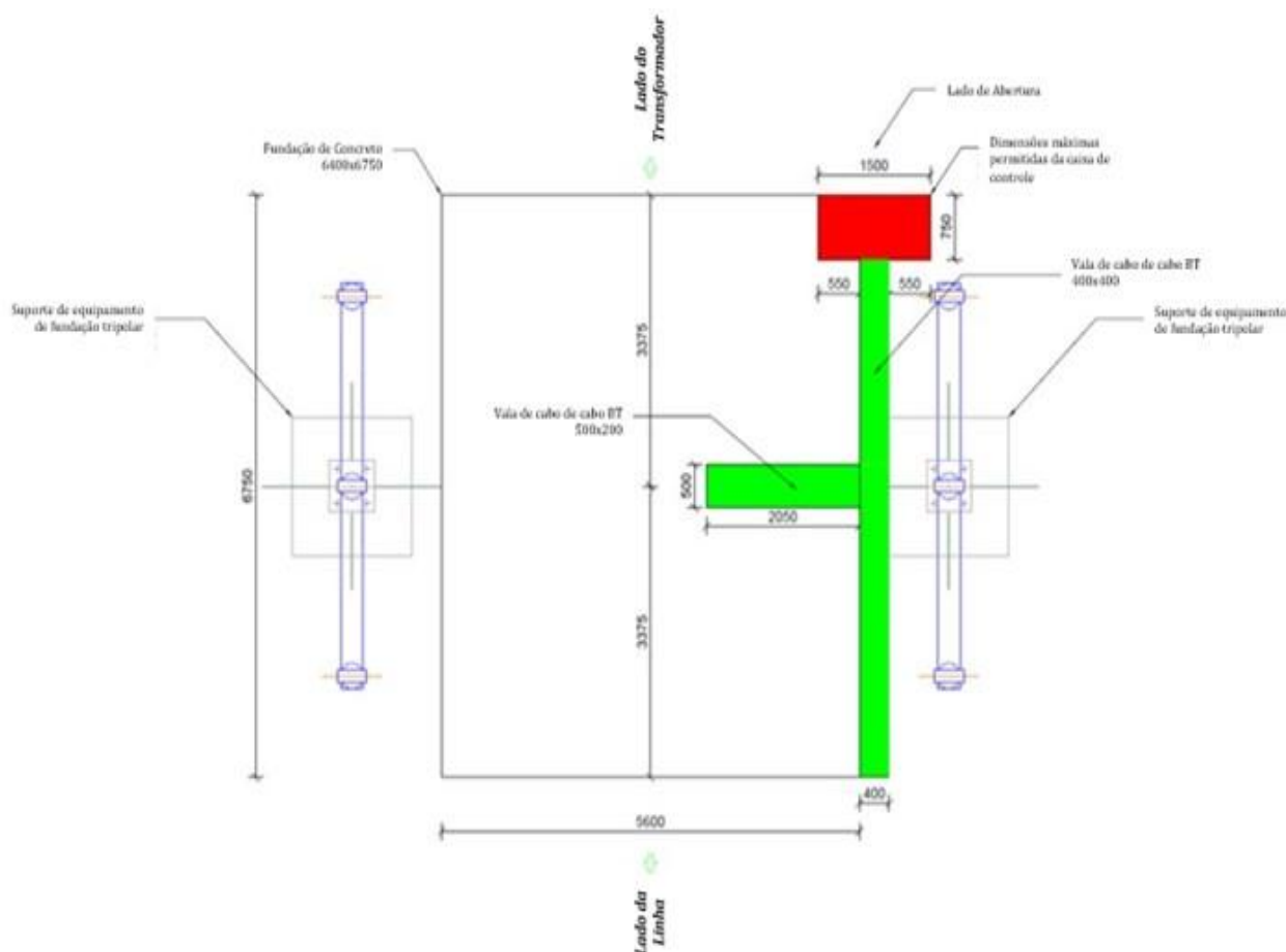
Figura 94 - Vista de planta geral Fundação do Módulo Híbrido
