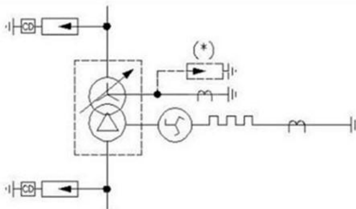
Figura 43 - Diagrama unifilar para conexão do resistor ao TFN
