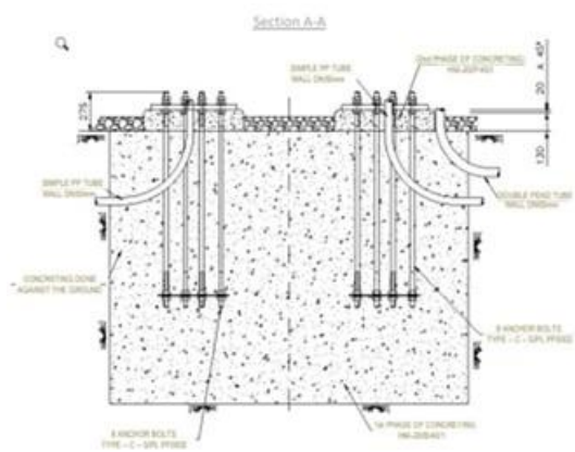
Figura 83 - Trecho AA da Pórtico Fundação
