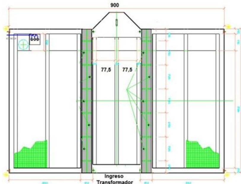
Figura 102 - Base do transformador de potência e recipiente de óleo
