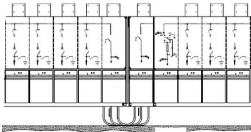
Figura 55 - Exemplo de interligação de módulos através de cabos
