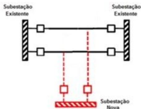
Figura 18 - Conexão em Derivação (Tap Dupla)
