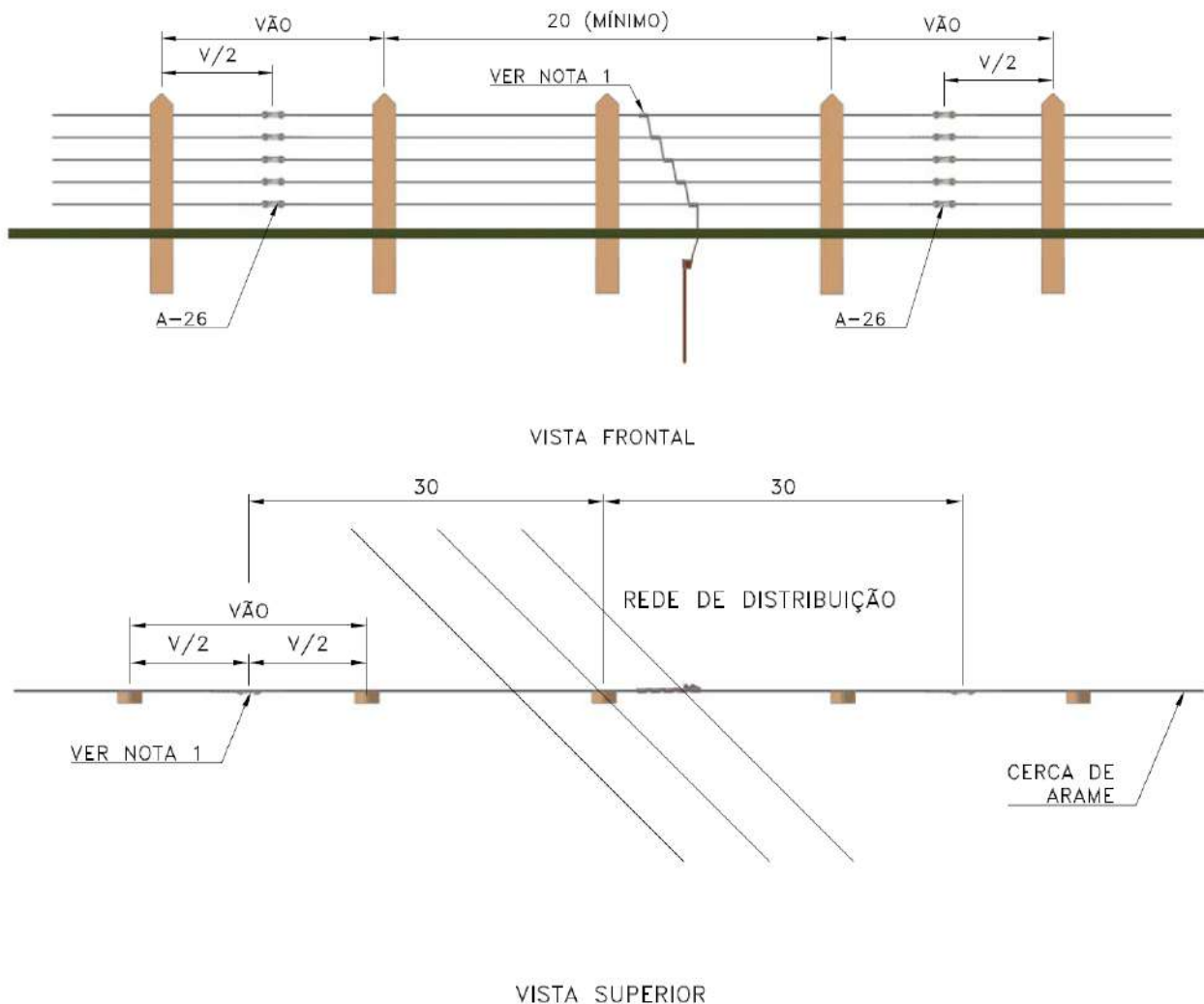
Desenho 7 – Seccionamento e aterramento de cercas transversais
