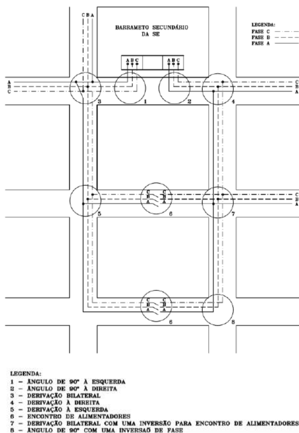
Figura 12 – Fases da rede primária
