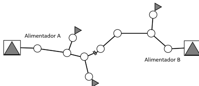
Figura 04 - Esquema radial com recurso
