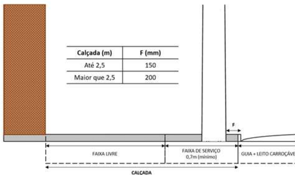
Figura 07 – Faixas de uso da calçada
