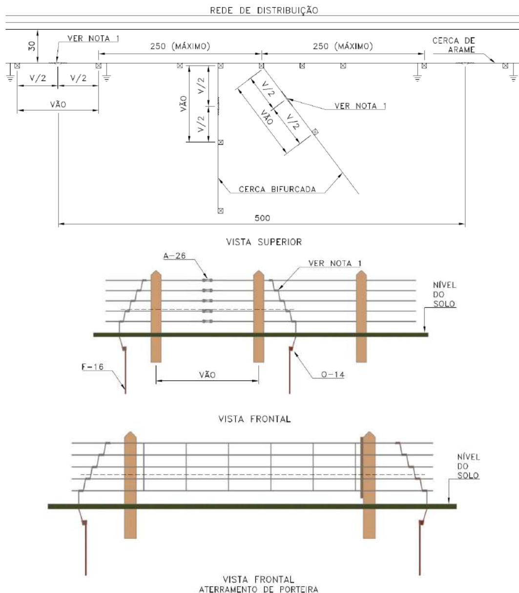
Desenho 6 – Seccionamento e aterramento de cercas paralelas e bifurcadas
