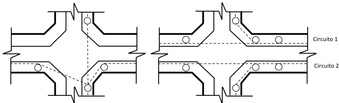
Figura 09 – Derivações em esquinas
