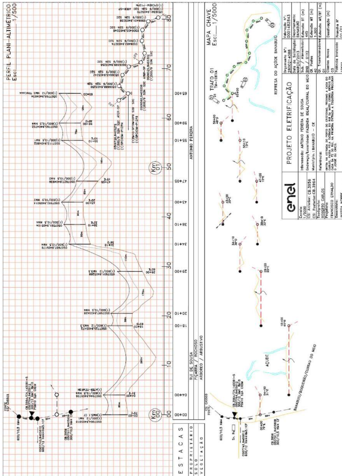
Desenho 14 – Perfil planialtimétrico
