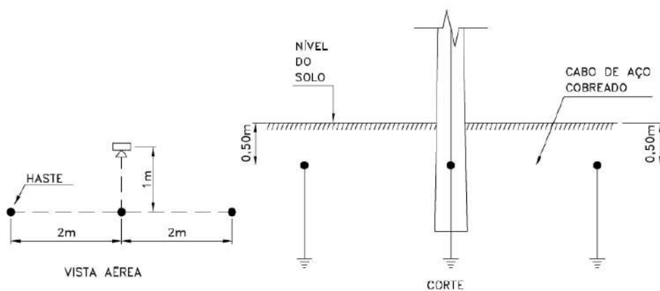
ATERRAMENTO COM 3 HASTES
