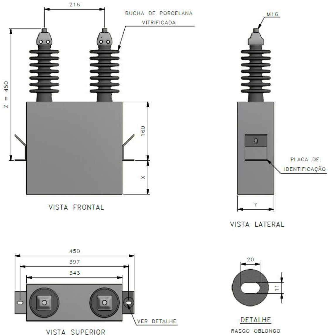
Figura 1 – Capacitor de Potência em Derivação
