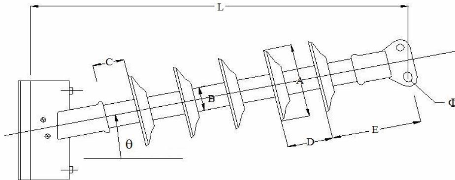
Figura 8: Aislador polimérico tipo line post (pilar). Terminación Drop-eye.
