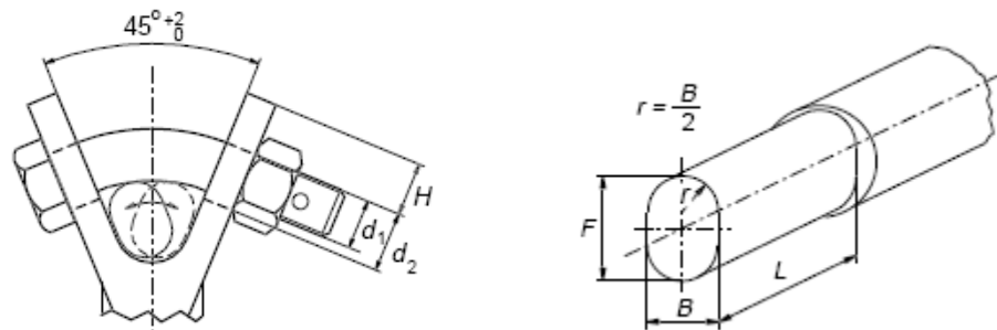
Figura 2: Acoplamiento tipo Y-clevis (IEC 61446-1)
