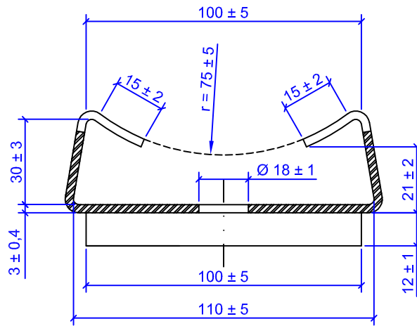
CORTE AB
