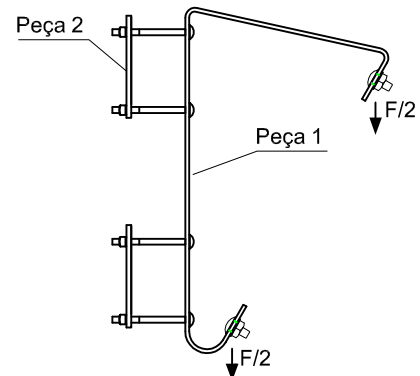
Montagem e detalhe de ensaio
