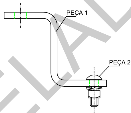
DETALHE DE MONTAGEM
