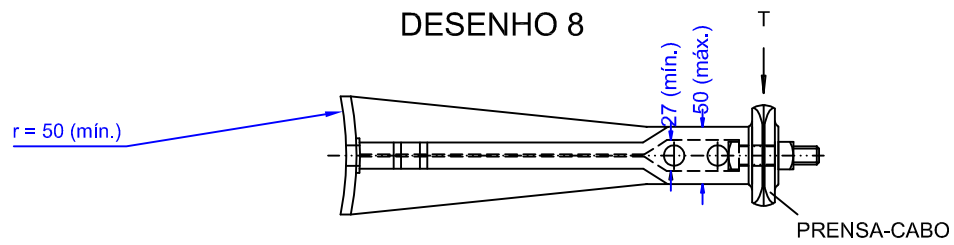
VISTA INFERIOR
