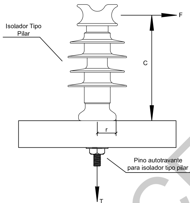
Item Código CELG D A (mm) B (mm) Diâmetro D 1 46487 38 38 M20 2 24414 140 80 3 46488 170 140 4 46489 200 140 5 46490 250 150 6 46491 300 150 7 46492 350 150
