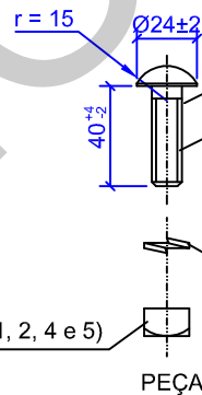
PEÇA 2
