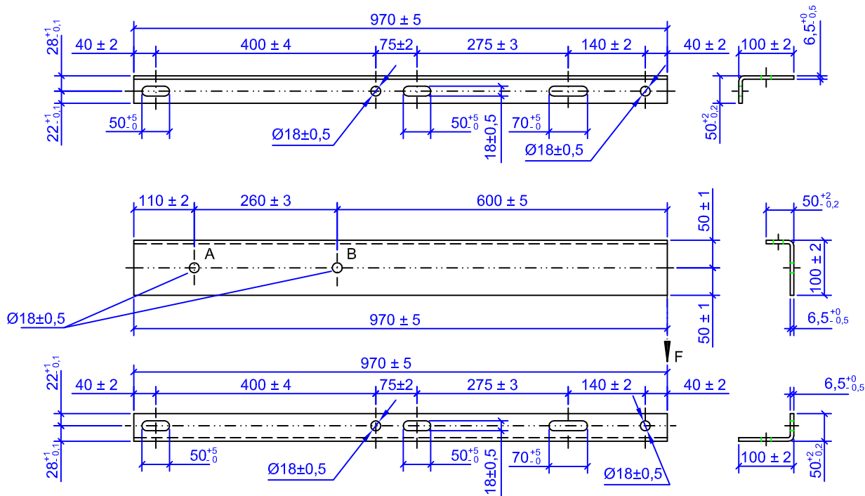
SUPORTE FD
