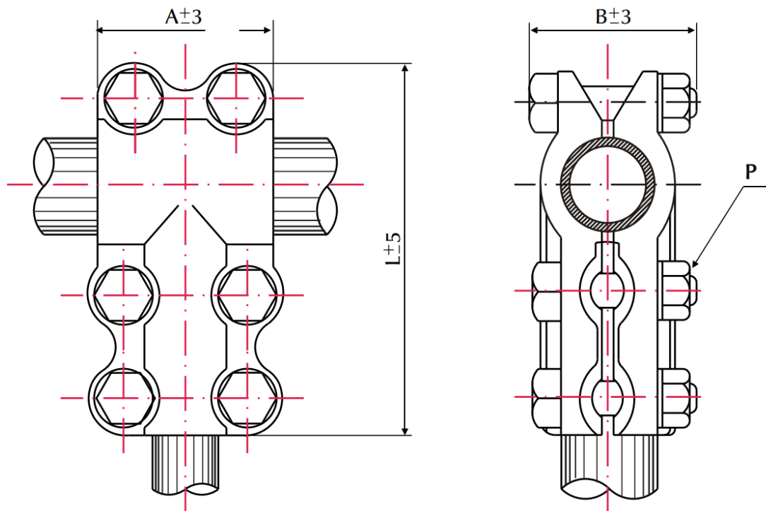
Figura 1 - Conector "T" Para Tubo de Alumínio ou Cobre no Tronco e na Derivação
