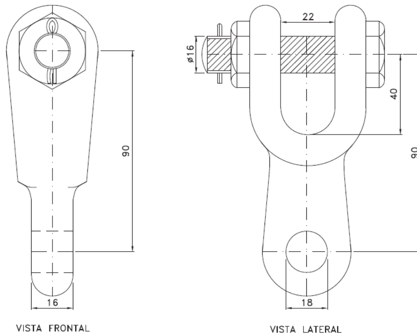
Figura 1 –Garfo-Olhal 90°
