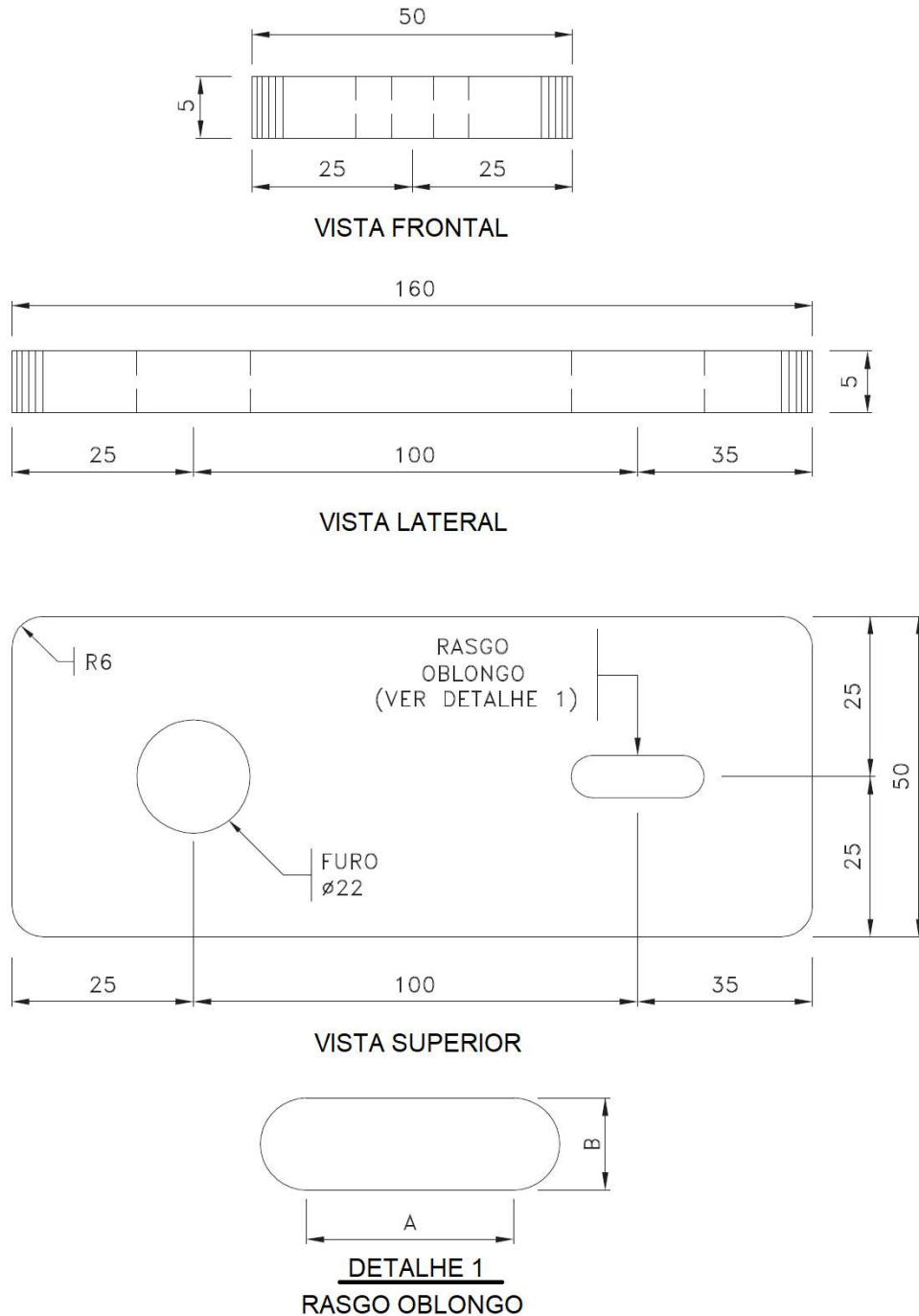
Figura 1 - Chapa Lisa para Aterramento
