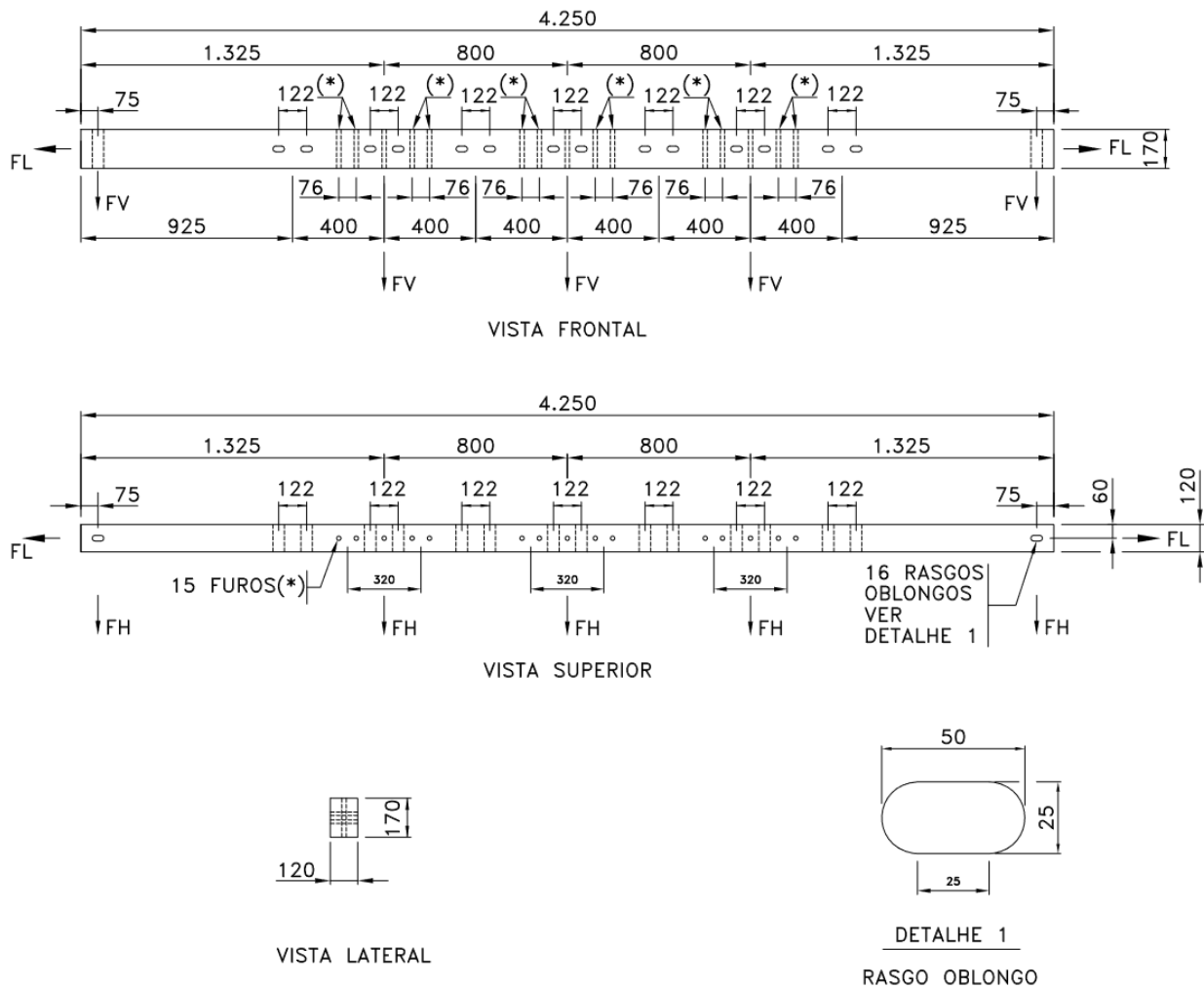
Figura 1 – Viga de Concreto Armado – Suporte para Seccionador Unipolar do Regulador de Tensão.
