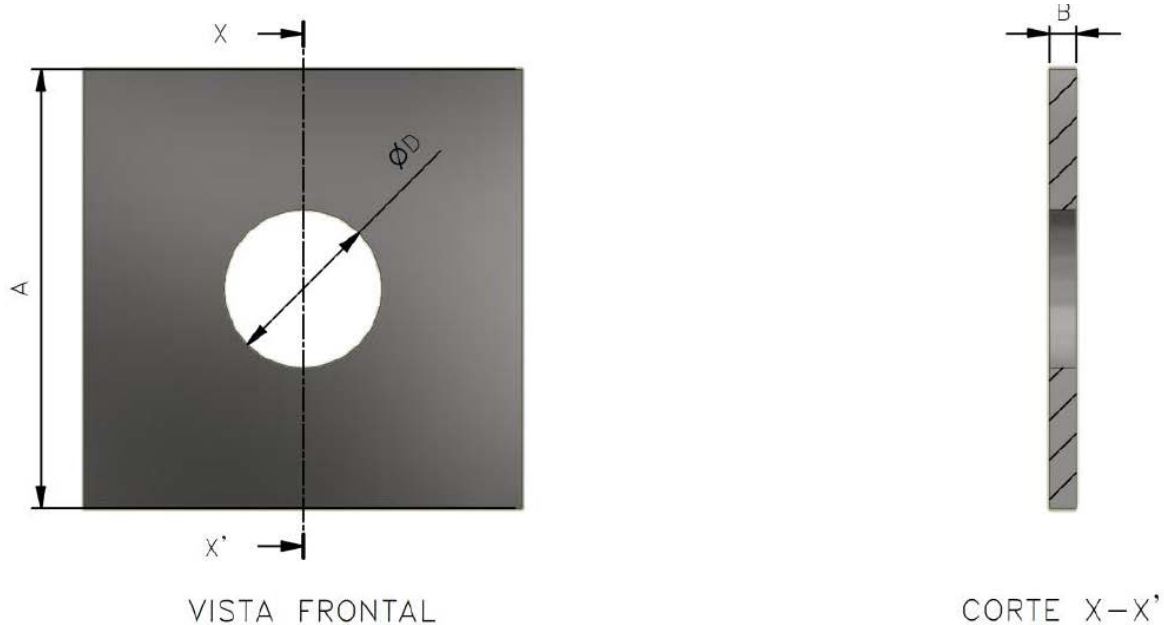
Figura 1 - Arruela Quadrada
