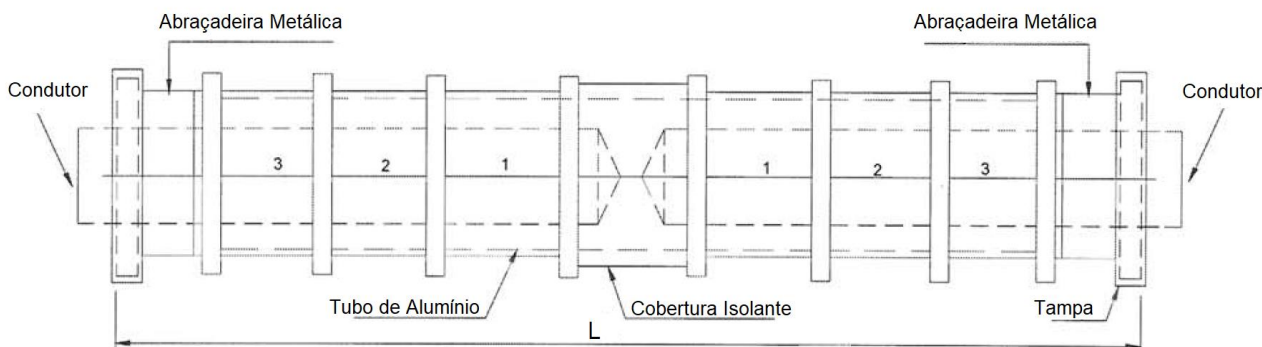
Figura 1 - Luva de Emenda Isolada para Cabo de Alumínio BT
