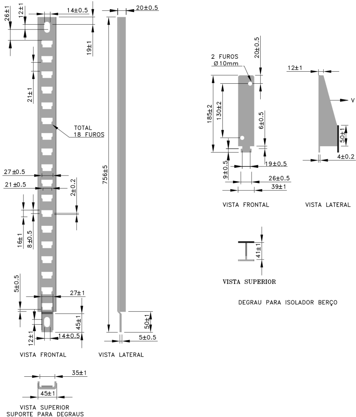
Figura 1 - Suporte para isolador berço
