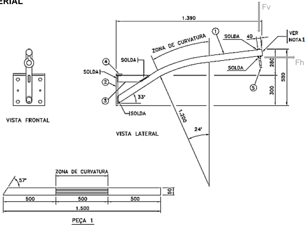
Figura 1 - Vistas e detalhes da peça
