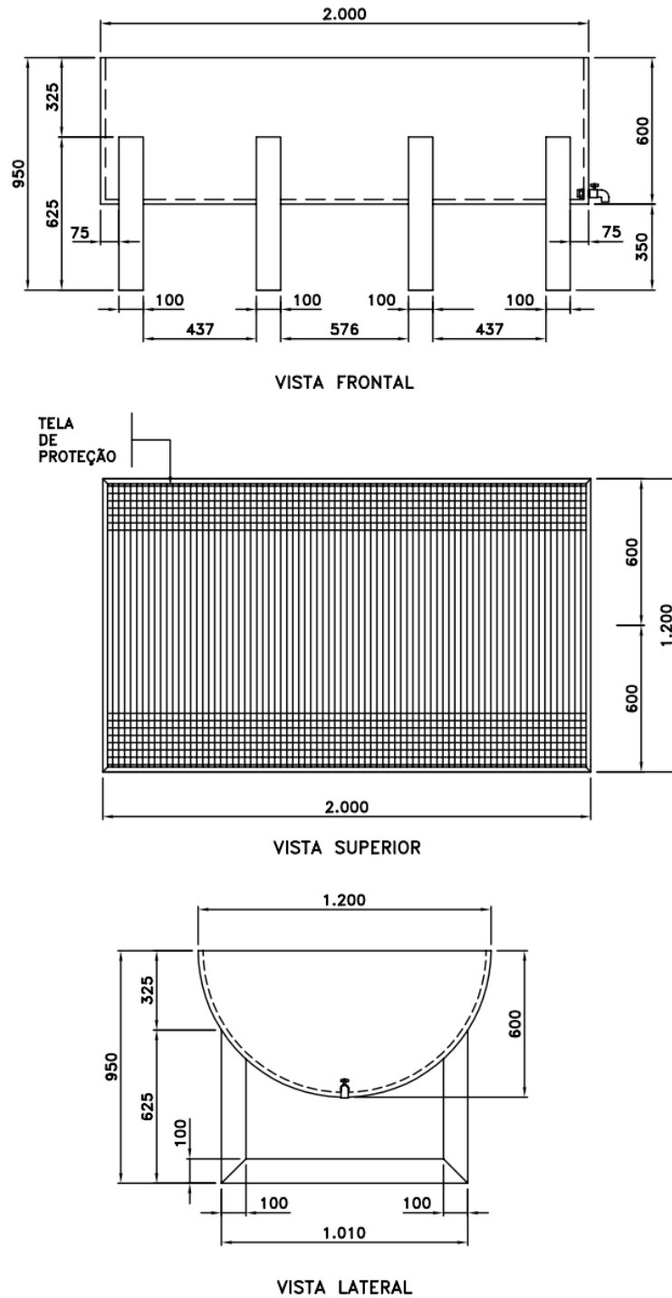
Figura 1 - Coletor Fixo para óleo de Transformador
