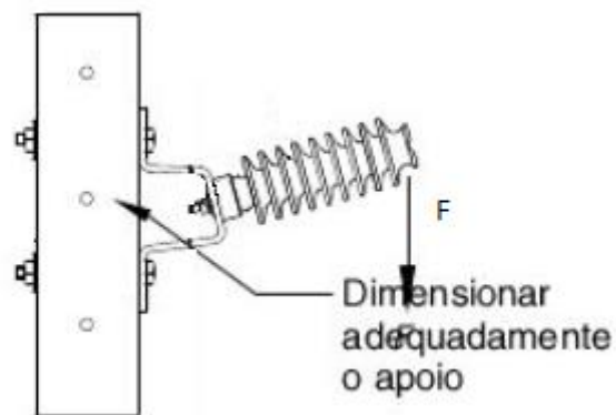
Figura 2 - Ensaio mecânico
