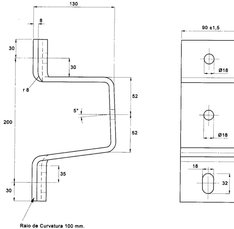
Figura 1 - Suporte Lateral
