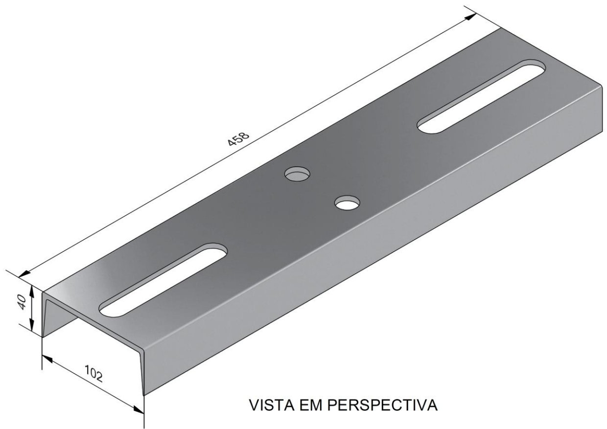
Figura 5 – Suporte para Instalação de Seccionadora Unipolar – Tipo 4
