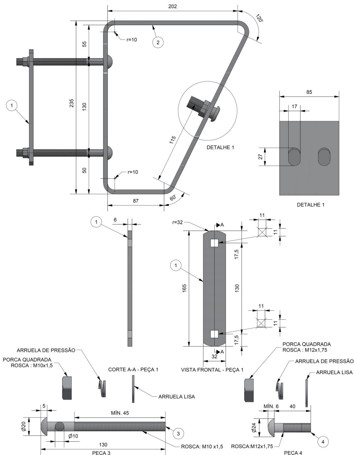
Figura 6 – Suporte para Instalação de Seccionadora Unipolar – Tipo 5
