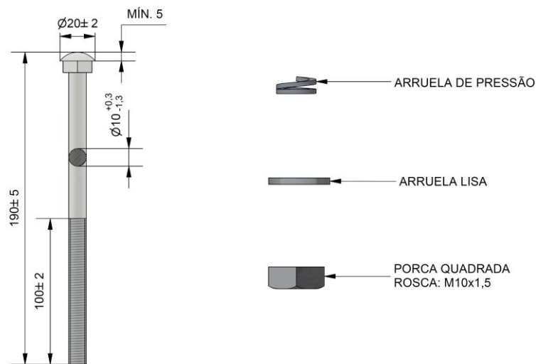
Figura 3 – Suporte para Instalação de Seccionadora Unipolar – Tipo 2
