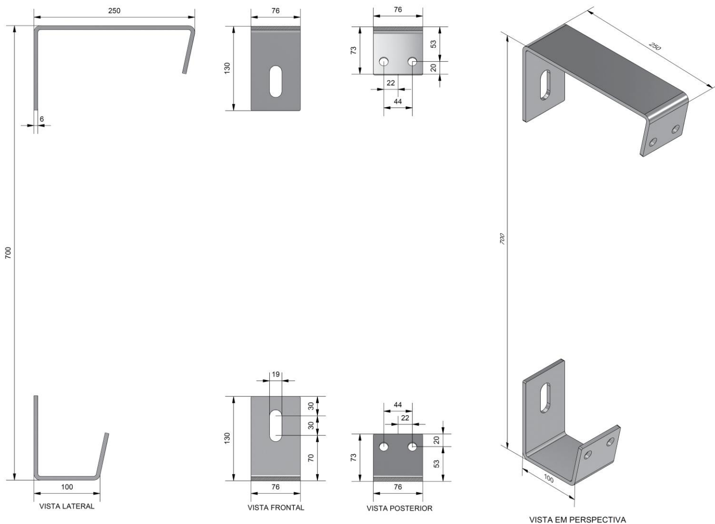
Figura 4 – Suporte para Instalação de Seccionadora Unipolar – Tipo 3
