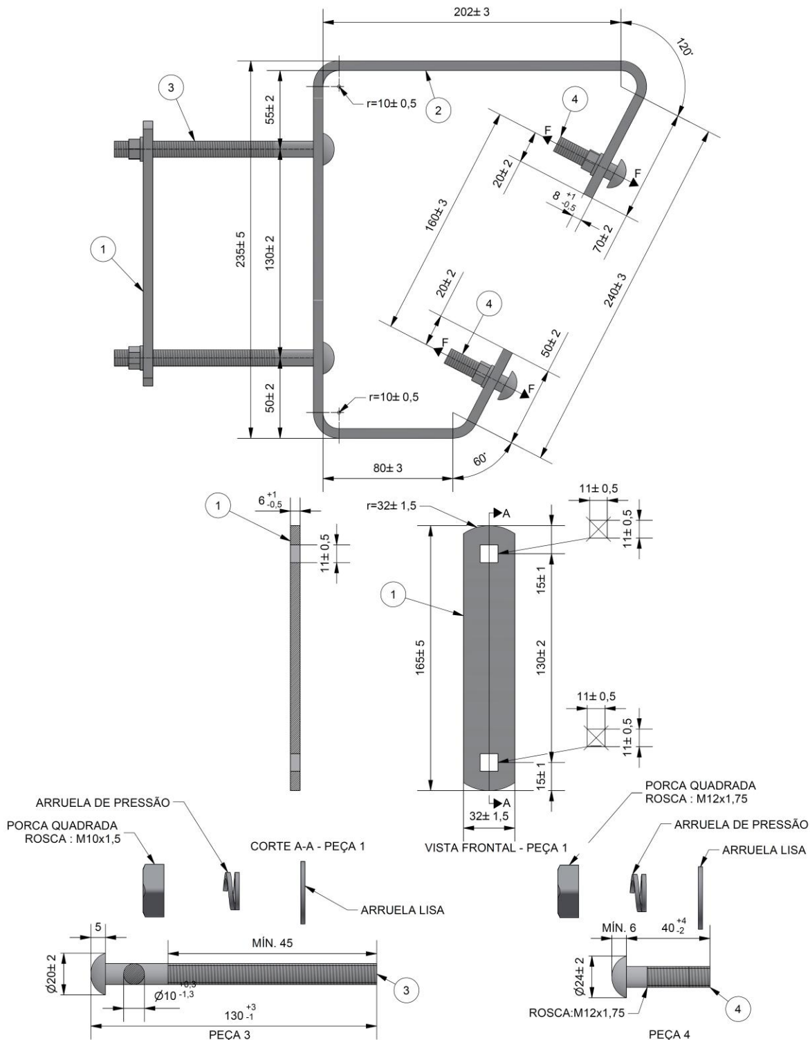
Figura 1 – Suporte para Instalação de Seccionadora Unipolar – Tipo 1
