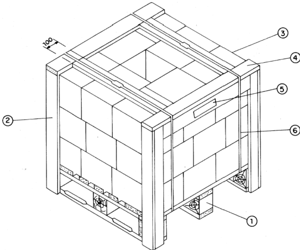
Figura 4 – Palete para transporte de medidores eletrônicos
