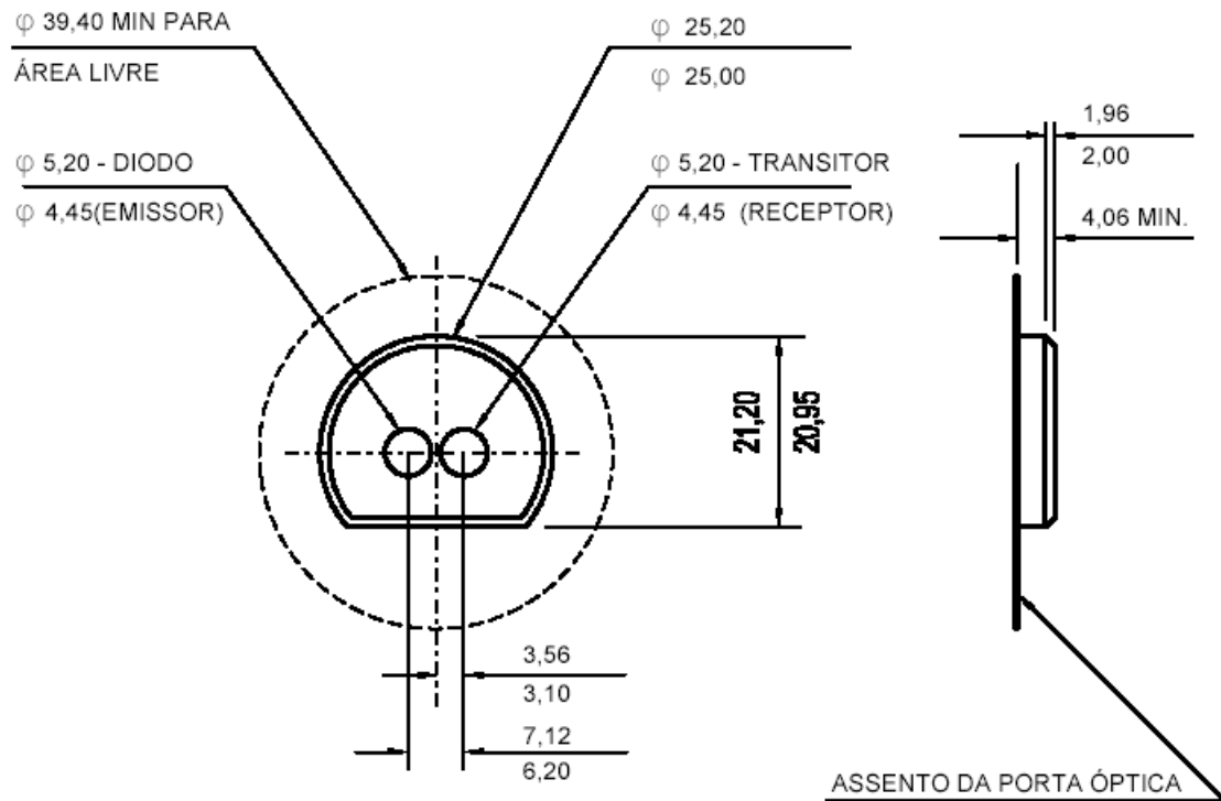
Figura 3 – Conector magnético da porta óptica
