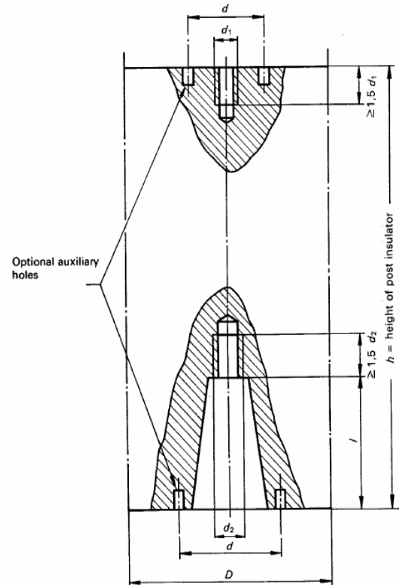
Figura 1: Aislador tipo soporte polimérico. 2
