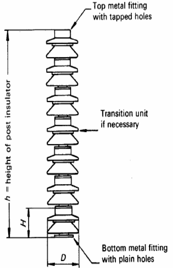
Figura 3: Aislador tipo pedestal.
